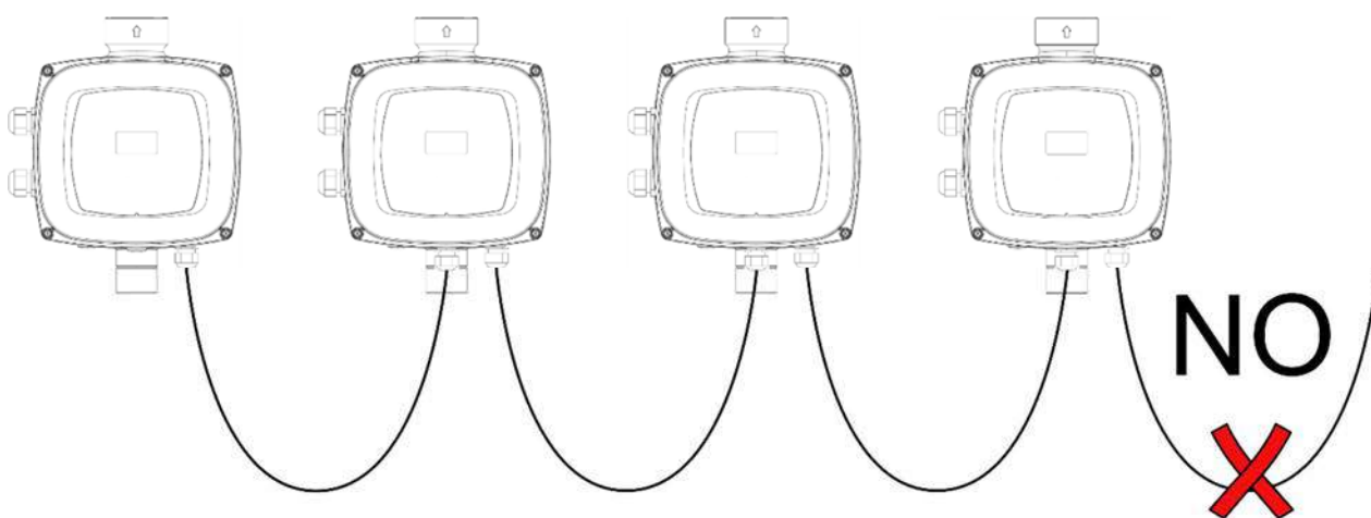
Σχήμα 9: Μην αφήνετε καλώδια συνδεδεμένα μόνο στο ένα άκρο
