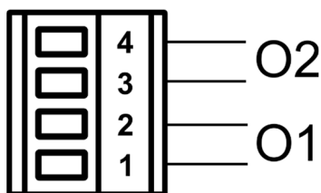
Abbildung 5: Anschluss der Ausgänge
