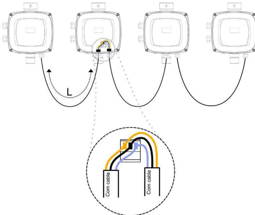
Afbeelding 6: Aansluitvoorbeeld van communicatie met meerdere inverters, met 4 apparaten
