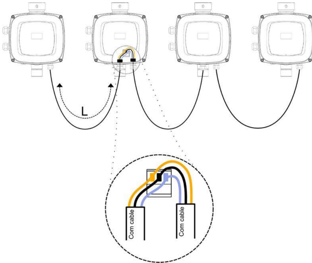
Figura 6: Exemplo de ligação da comunicação multi inversor com 4 dispositivos
