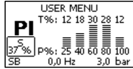
Şekil 15: Güç histogramı
