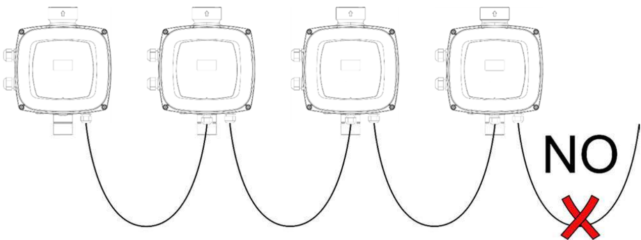
Abbildung 9: Keine nur an einem Ende angeschlossenen Kabel belassen
