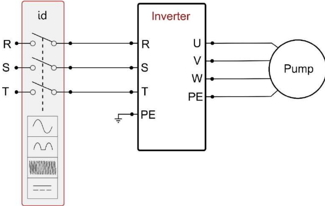
Şekil 3b: Trifaze besleme ile kurma örn
