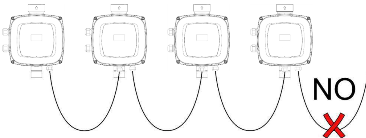
Figura 9: Non lasciare cavi connessi ad una sola estremità
