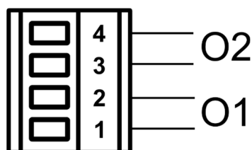
Figura 5: Conexión de las salidas
