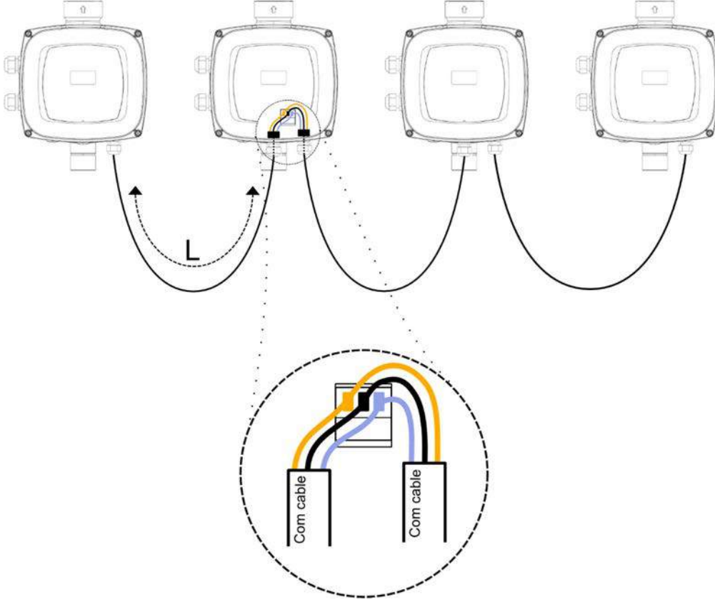
Şekil 6: 4 aygıtlı multi inverter haberleşmenin bağlantı örneği
