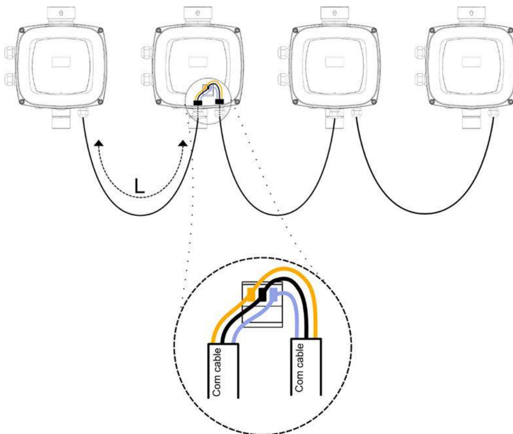
Obr. 6: Příklad připojení komunikace multi inverter se 4 zařízeními
