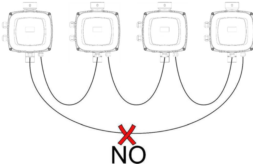
Abbildung 7: Keine Schleifenschaltung herstellen
