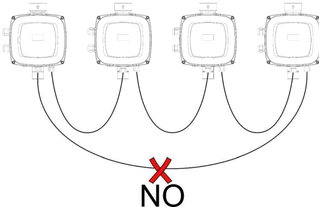
Figure 7: Ne pas effectuer de branchements en boucle
