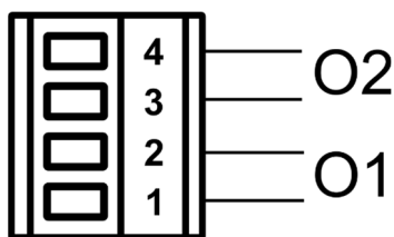
Figure 5: Connexion des sorties
