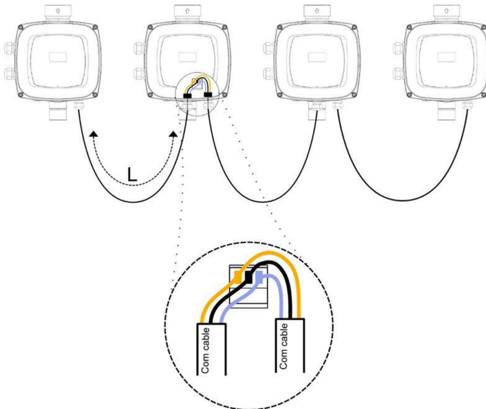
Figura 6: Esempio di connessione della comunicazione multi inverter con 4 dispositivi
