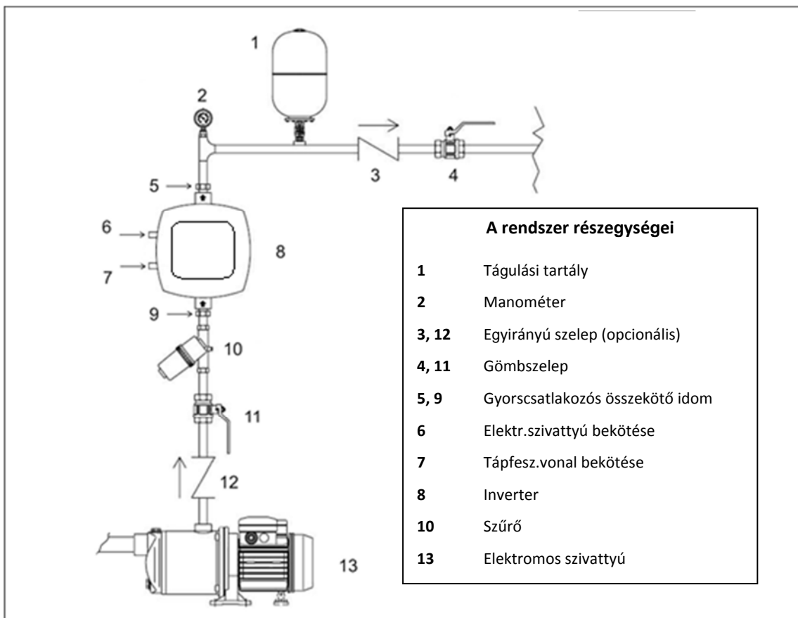
1. Ábra: Hidraulikus installáció
