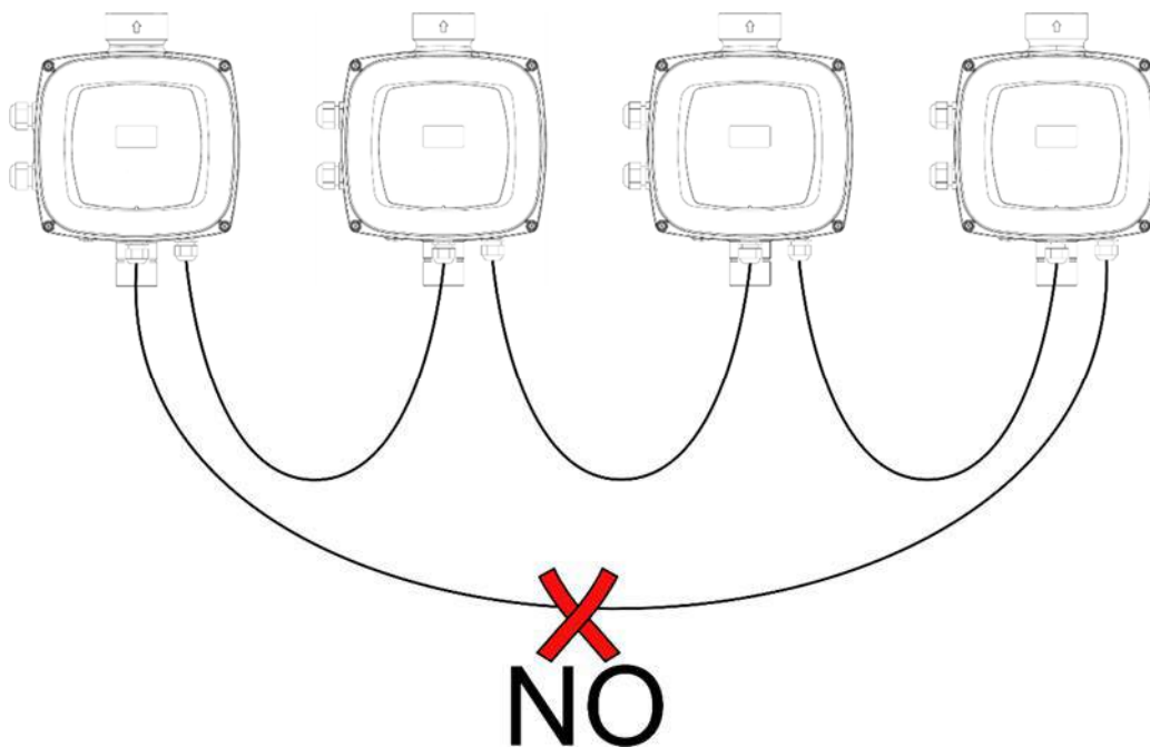
Afbeelding 7: Geen lusaansluitingen maken
