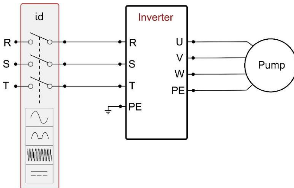
Rysunek 3b: Przykład zainstalowania z zasilaniem trójfazowym
