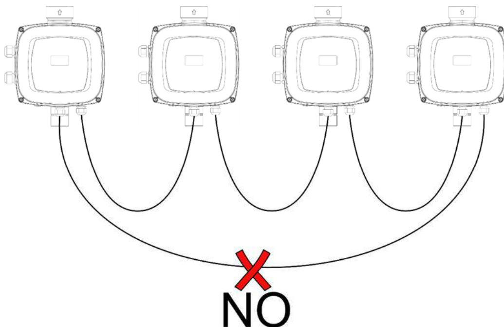
Σχήμα 7: Μην κάνετε σύνδεση δακτυλίου
