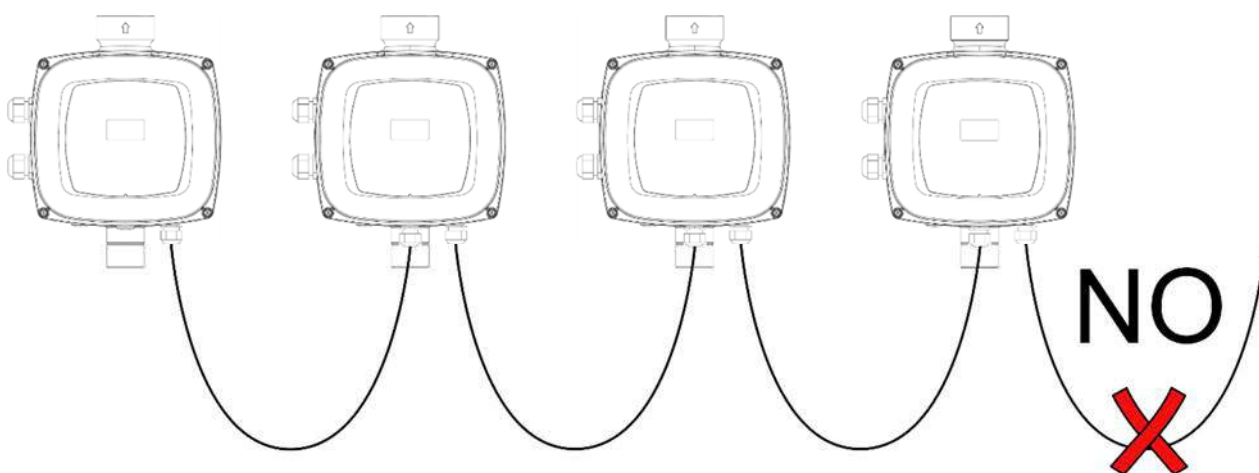
Afbeelding 9: Geen kabels aangesloten laten aan één uiteinde
