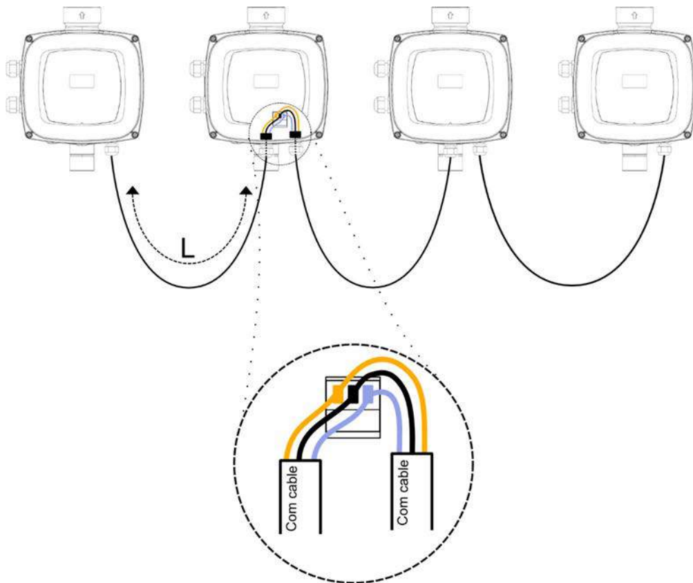
Fig. 6: Exempel på anslutning för kommunikation mellan flera inverterar med fyra anordningar
