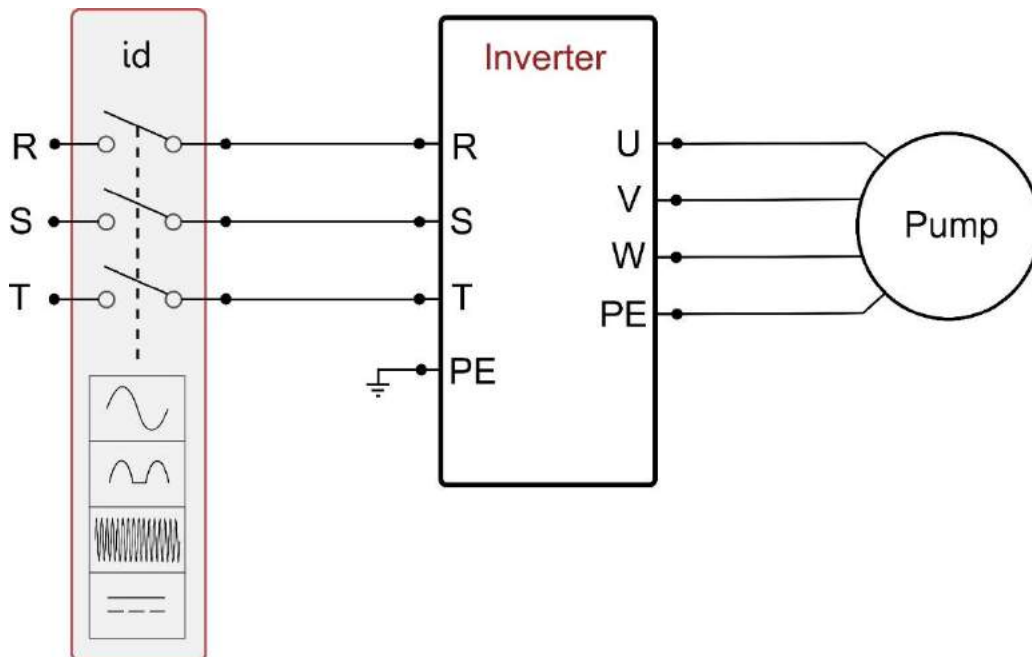
Σχήμα 3β: Παράδειγμα εγκατάστασης με τριφασική τροφοδοσία
