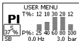
Rysunek 15: Histogram mocy
