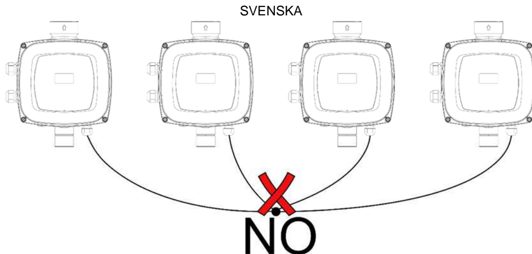
Fig. 8: Utför inte stjärnanslutningar
