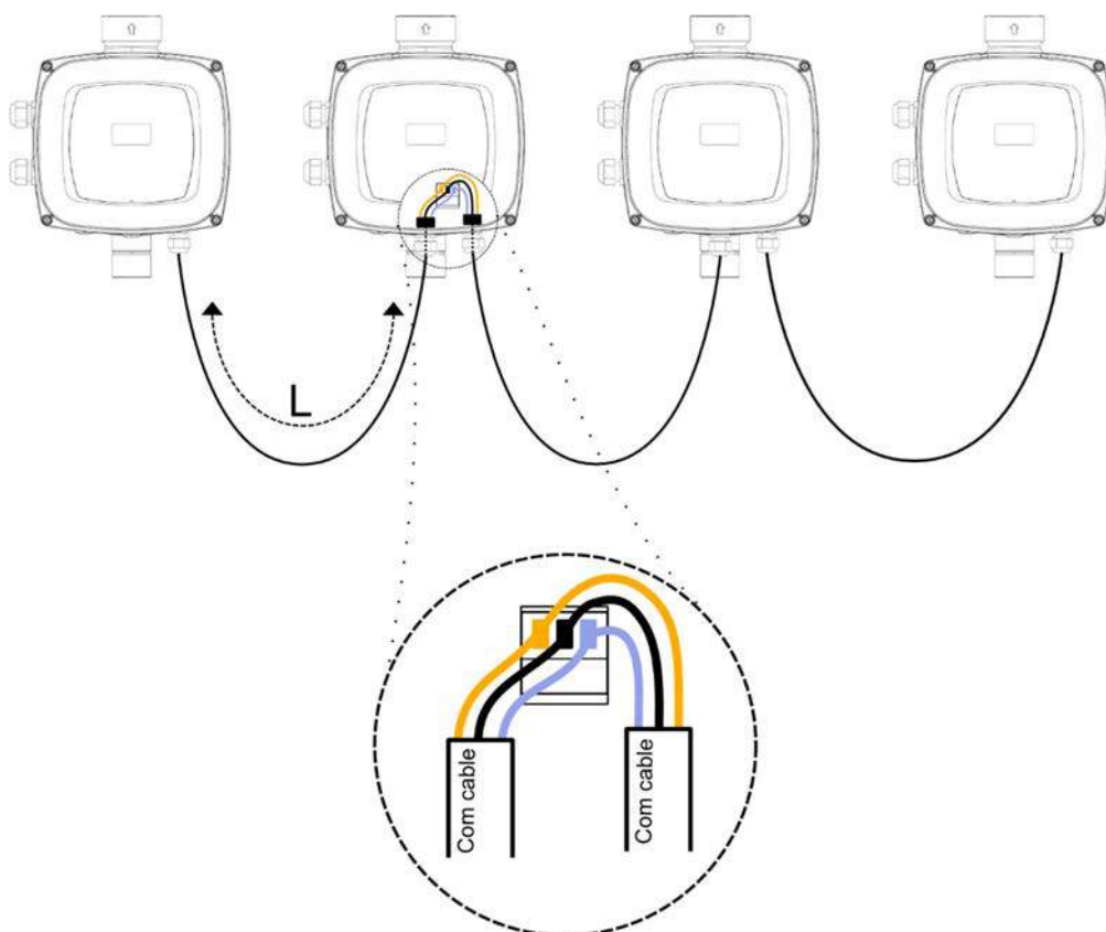
Obrázok 6: Príklad pripojenia komunikácie pre multi inverter so 4 zariadeniami
