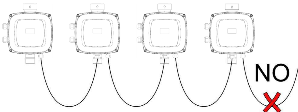
Figura 9: Não deixar cabos ligados a uma só extremidade
