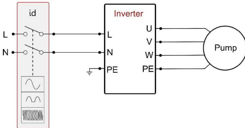
Σχήμα 2α: Παράδειγμα εγκατάστασης με μονοφασική τροφοδοσία
