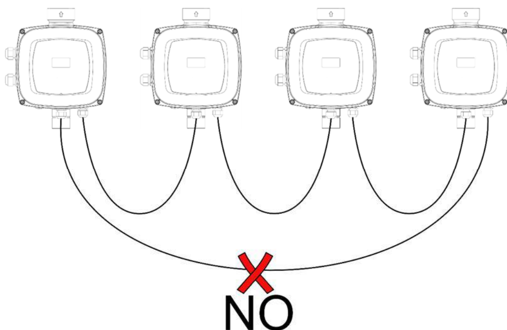
Obrázok 7: Nevykonávať prstencové spojenia
