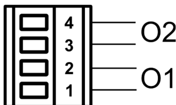
5. Ábra: A kimenetek bekötése
