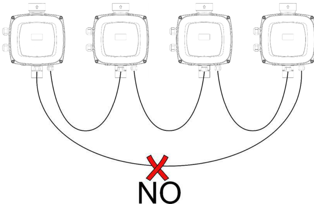
Kuva 7: Älä tee silmukkakytkentöjä
