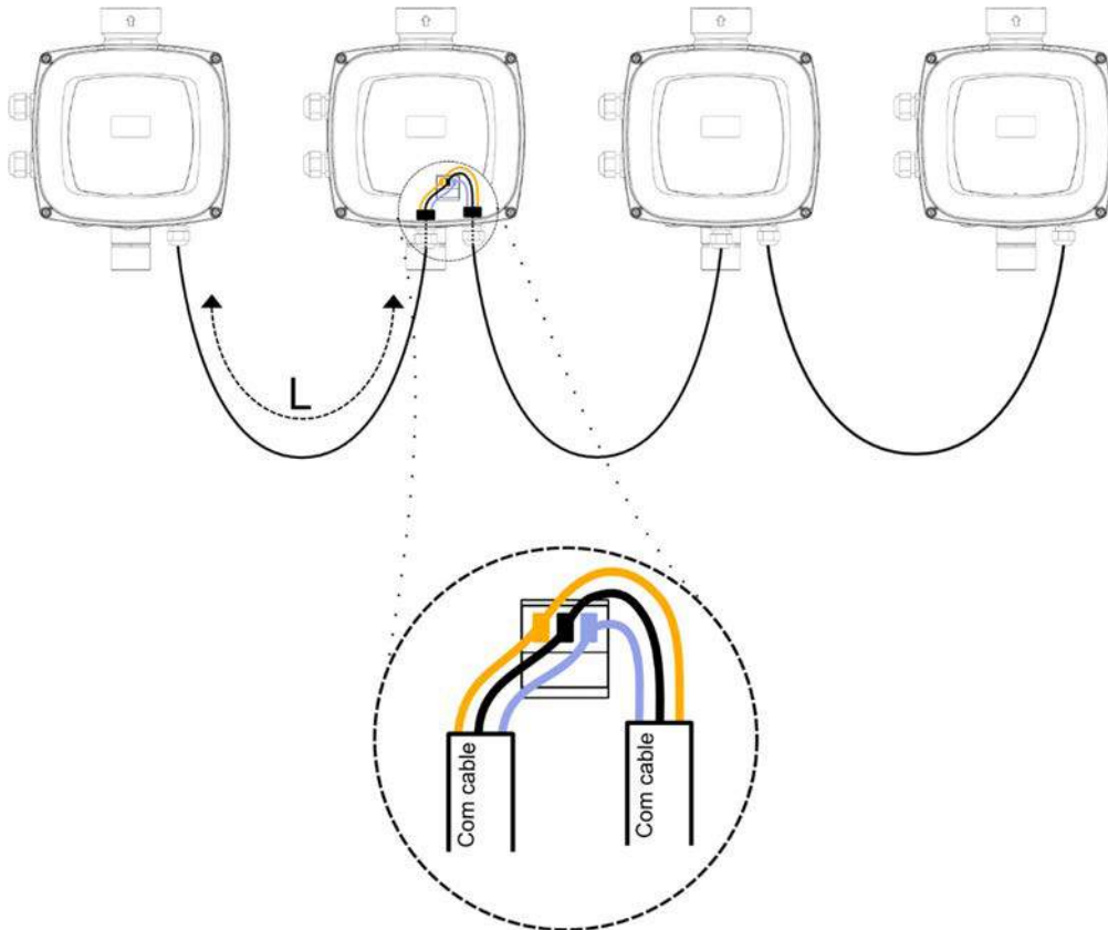
Abbildung 6: Beispiel für den Anschluss der Kommunikation Multi-Inverter mit 4 Geräten
