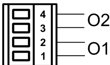
Obr. 5: Připojení výstupů
