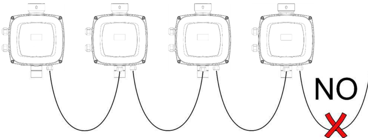
Figura 9: No dejar cables conectados solo a un extremo
