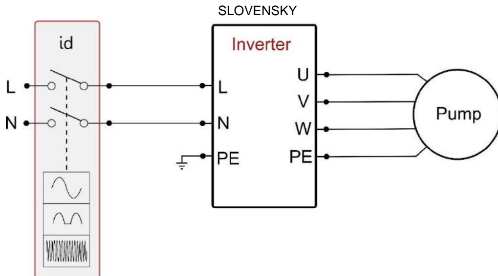
Obrázok 2a: Príklad inštalácie s jednofázovým napájaním
