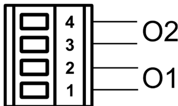
Kuva 5: Lähtöliitäntä
