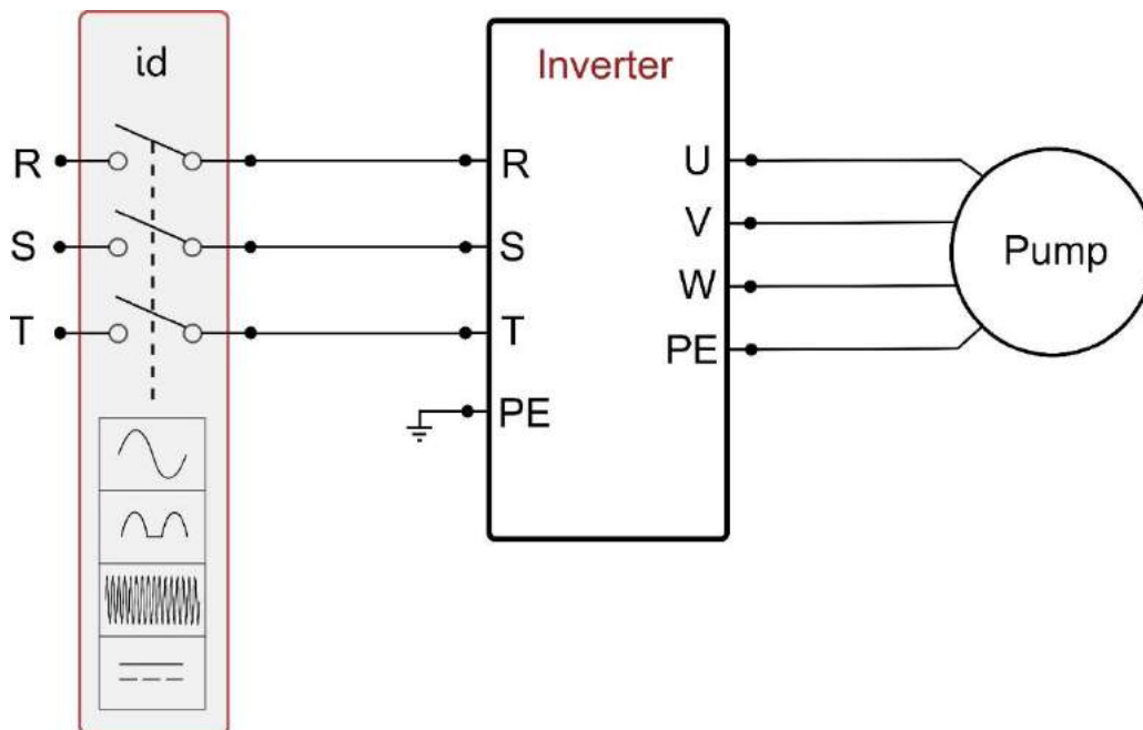
Малюнок 3b: Приклад встановлення за трифазного живлення
