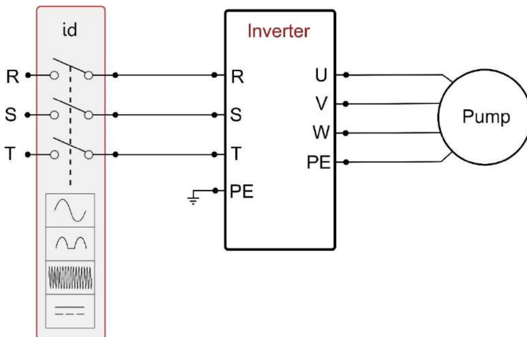
Fig. 3b: Exempel på installation med trefasmatning
