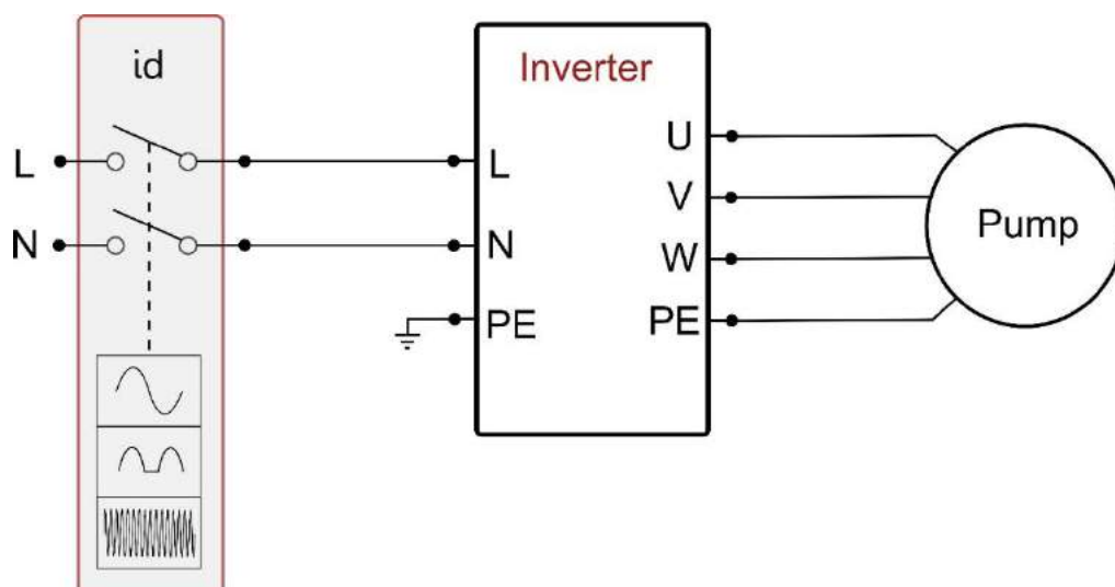
Rysunek 2a: Przykład zainstalowania z zasilaniem jednofazowym
