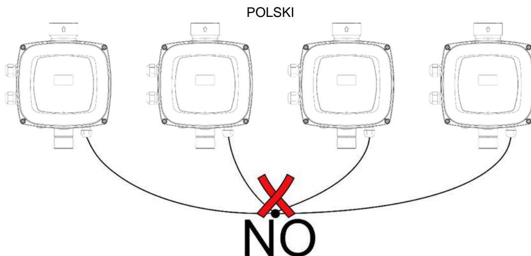
Rysunek 8: Nie wykonywać połączeń na gwiazdę
