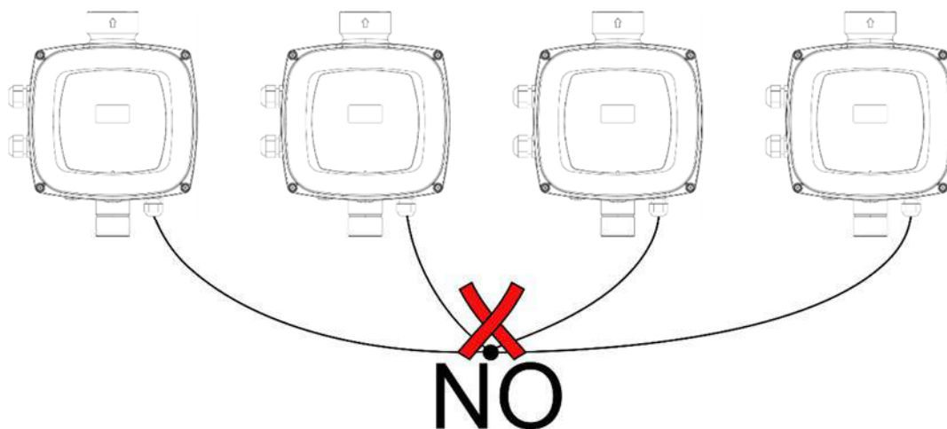
Figura 8: Non eseguire connessioni a stella
