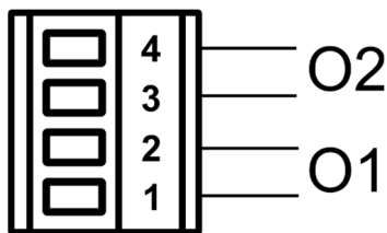
Rysunek 5: podłączenie wyjść
