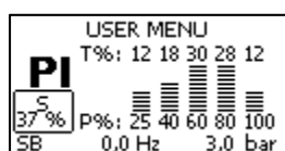
Figure 15: Histogramme de puissance
