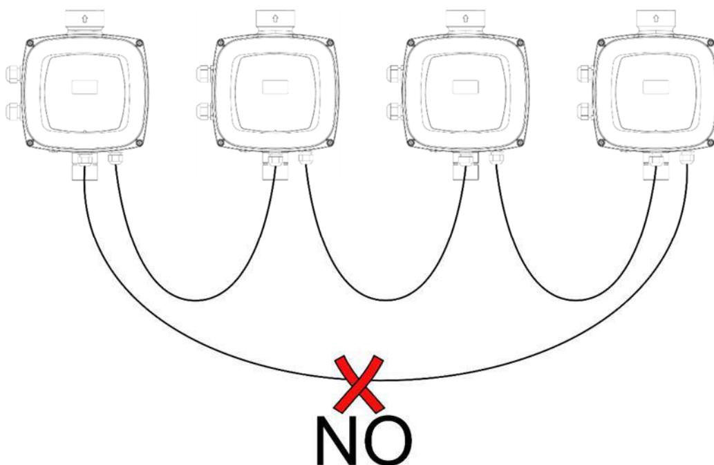
Figura 7: No realizar conexiones de anillo
