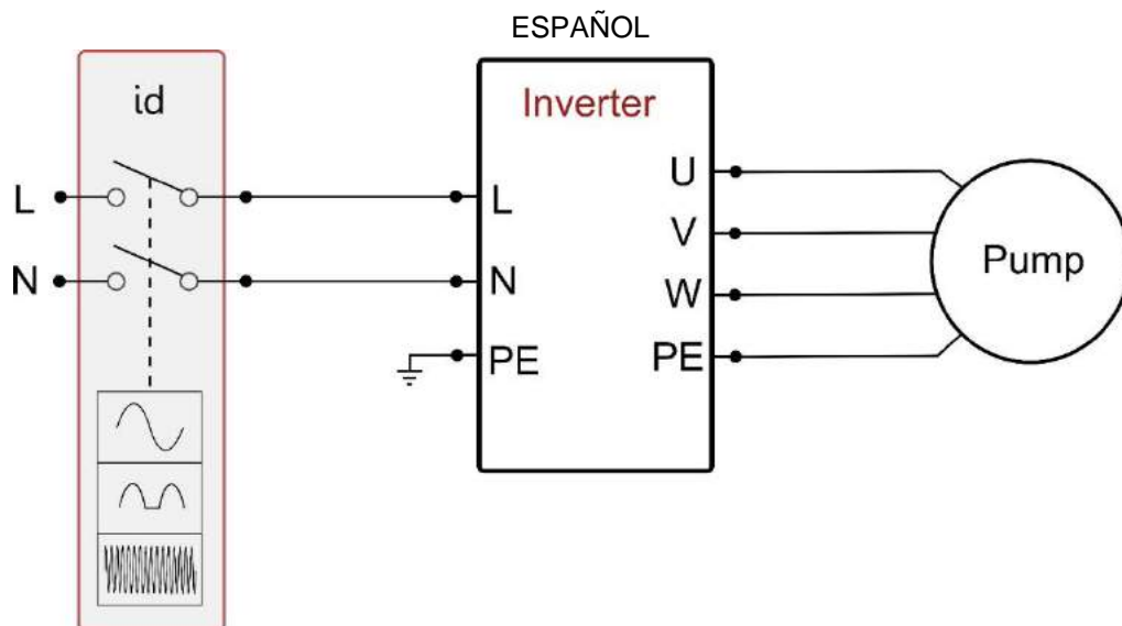
Figura 2a: Ejemplo de instalación con alimentación monofásica
