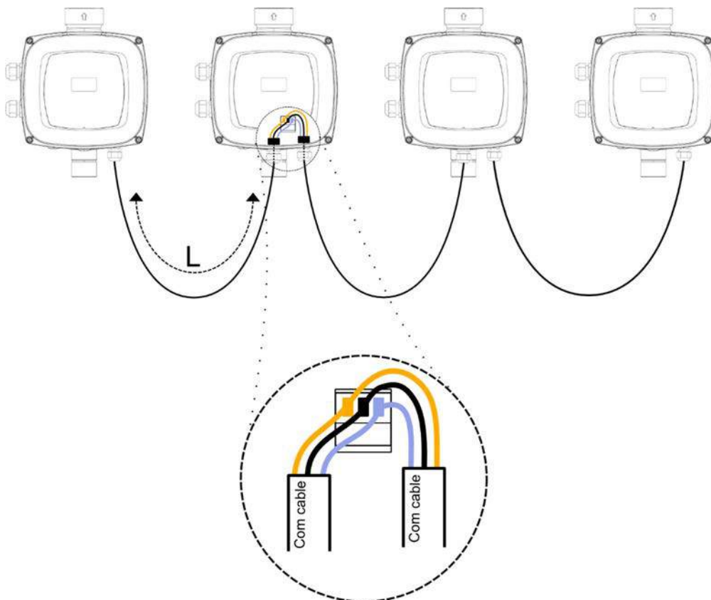
Figura 6: Ejemplo de conexión de la comunicación multi inverter con 4 dispositivos
