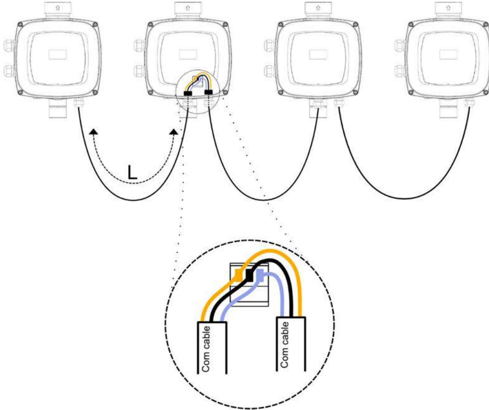
Σχήμα 6: Παράδειγμα συνδεσμολογίας της επικοινωνίας πολλαπλών αναστροφών με 4 συσκευές
