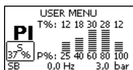
Σχήμα 15: Ιστόγραμμα ισχύος
