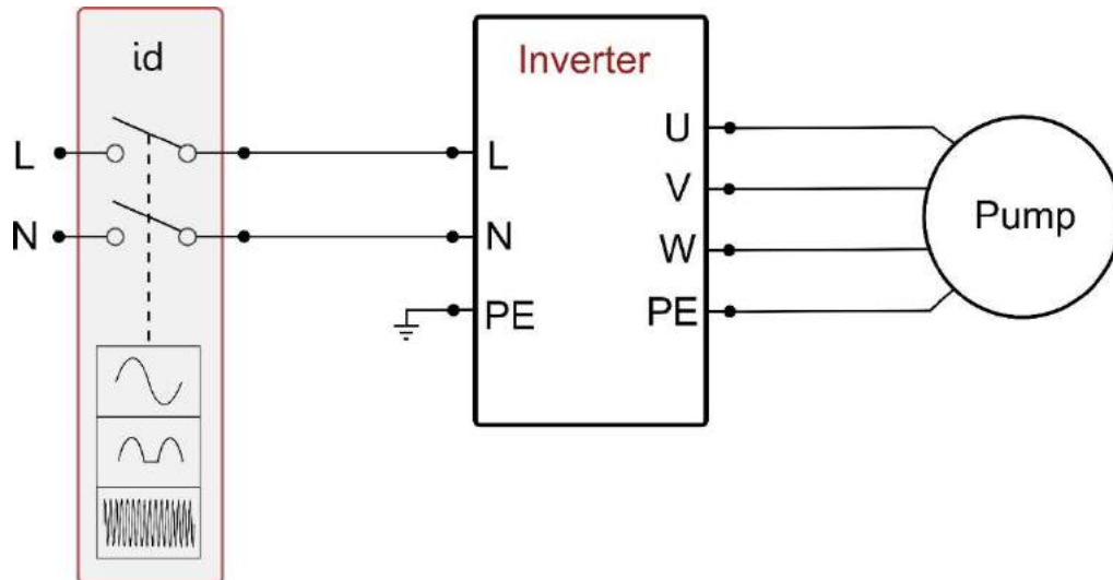
Abbildung 2a: Beispiel einer Installation mit Einphasenversorgung
