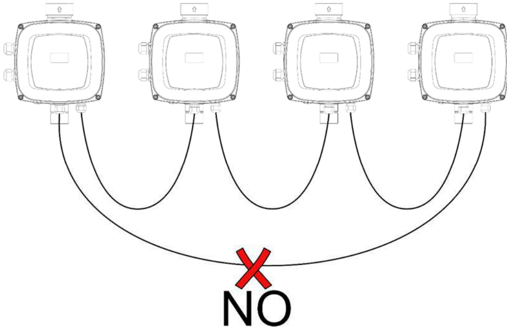
Şekil 7: Halka bağlantılar gerçekleştirilmeyiniz
