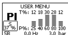
Figura 15: Histograma puterii
