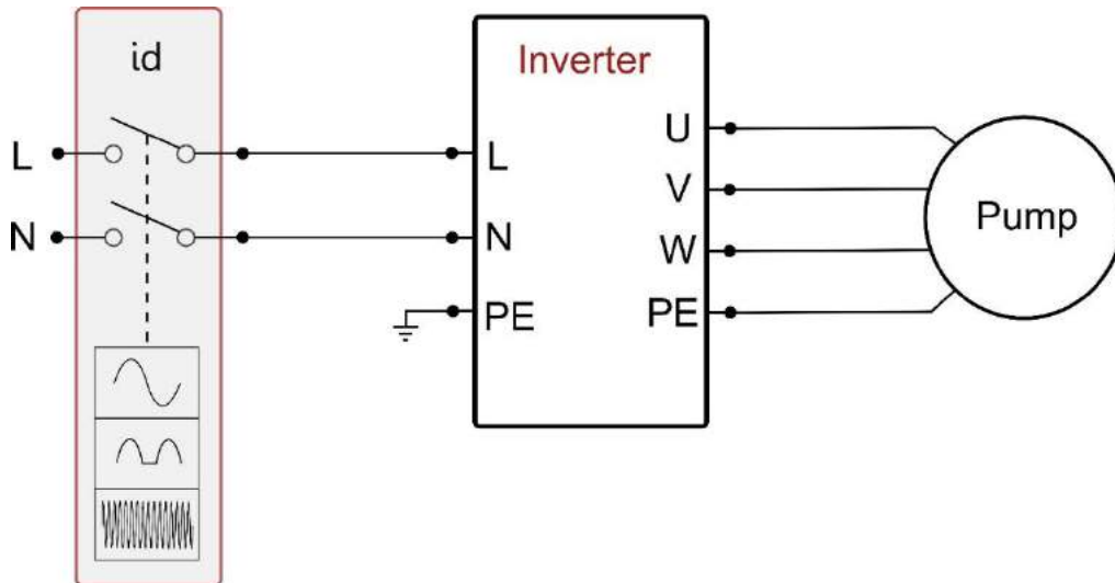
2a.: Ábra Installációs példa monofázisos ellátás esetén
