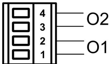
Obrázok 5: Pripojenie výstupov
