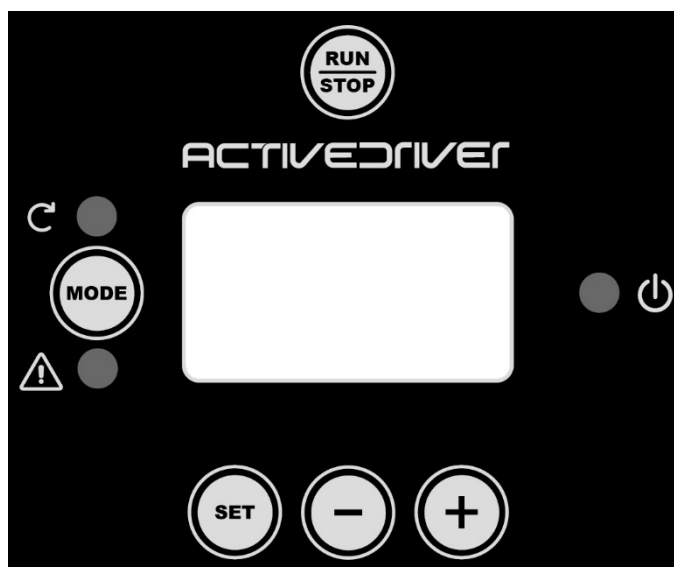
Kuva 11: Käyttöliittymän ulkomuoto
