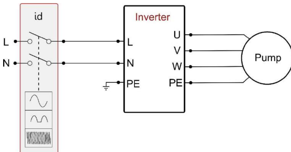
Fig. 2a: Exempel på installation med enfasmatning
