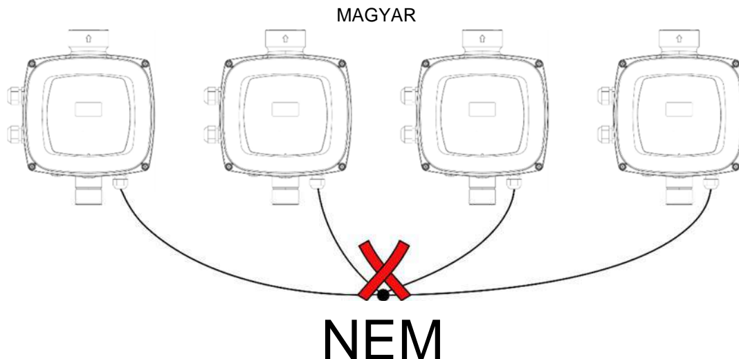
8. Ábra: NE végezzen csillag jellegű összekötéseket
