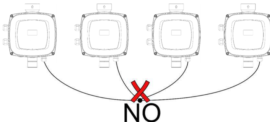
Figure 8: Ne pas effectuer de branchements en étoile
