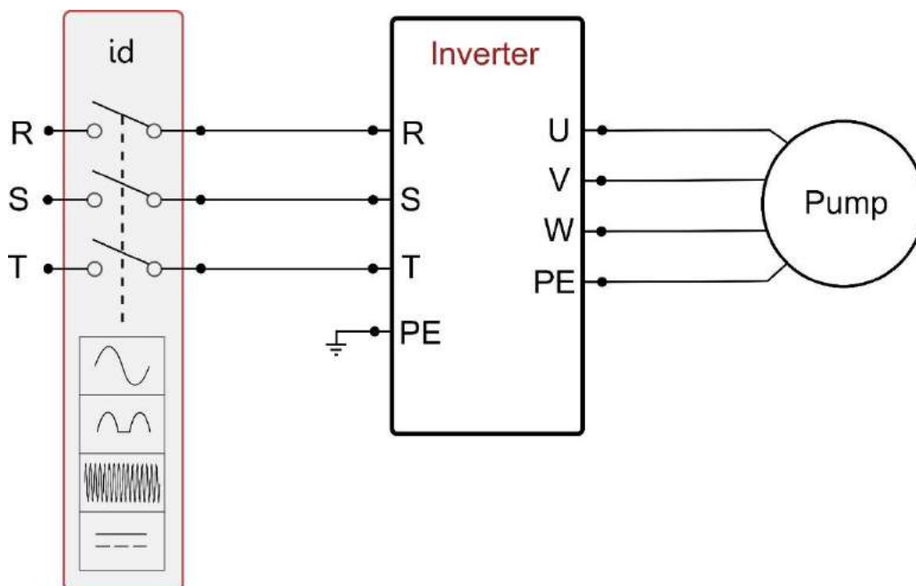
Figura 3b: Esempio di installazione con alimentazione trifase
