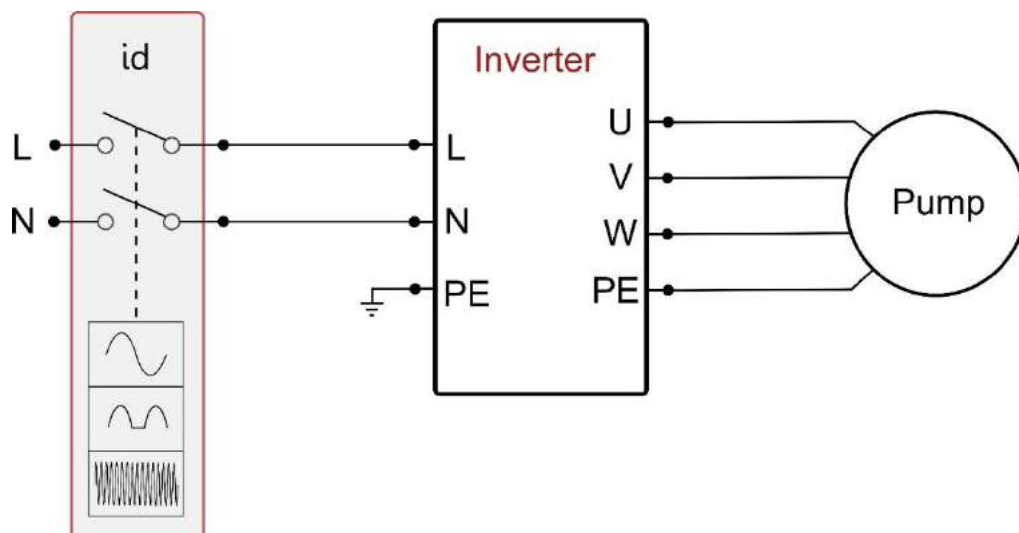
Obr. 2a: Příklad montáže s monofázovým napájením
