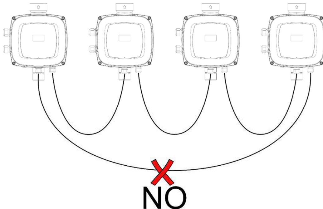
Fig. 7: Utför inte ringanslutningar
