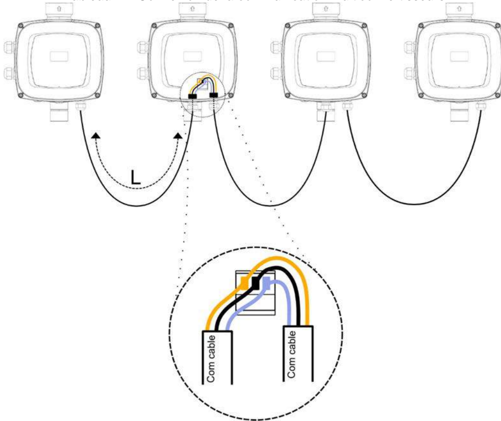
Figure 6: Exemple de branchement de la communication à inverseurs multiples avec 4 dispositifs
