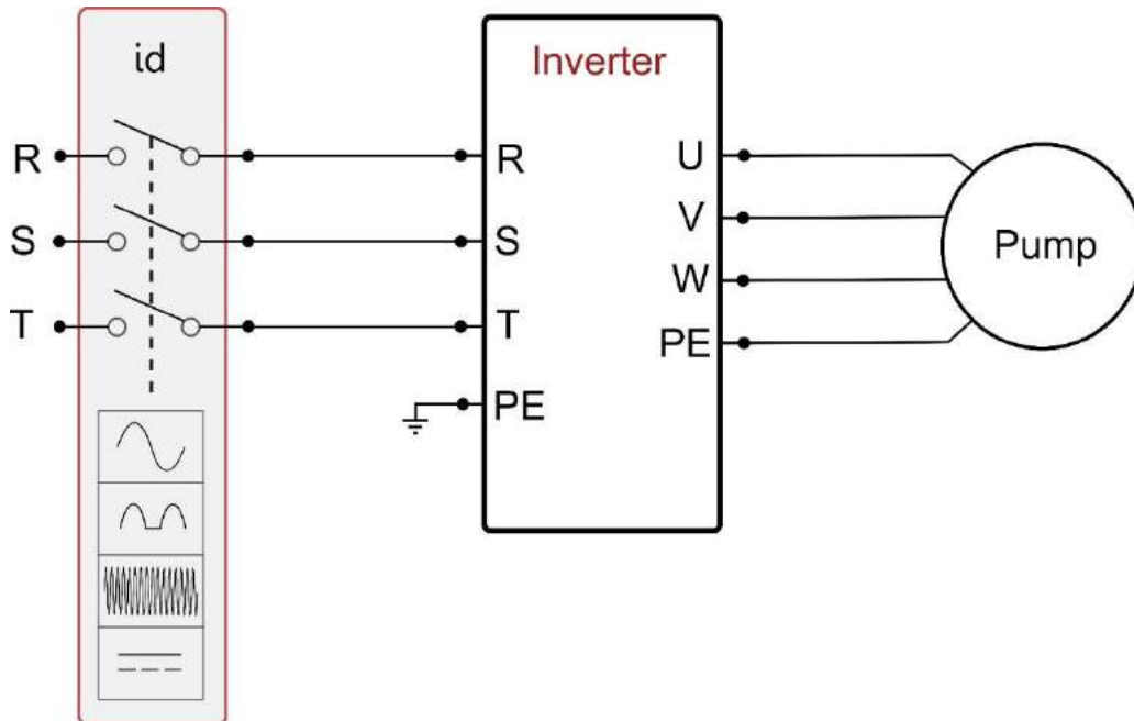
Figura 3b: Exemplo de instalação com alimentação trifásica
