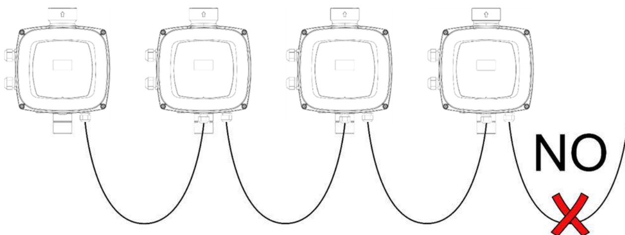
Fig. 9: Lämna inte kablar anslutna i bara ena änden
