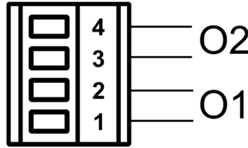
Şekil 5: Çıkışların bağlantısı
