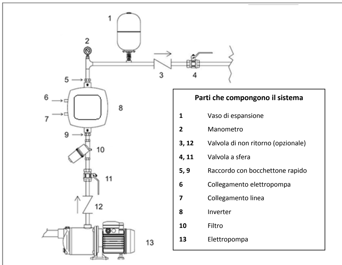
Figura 1: Installazione idraulica
