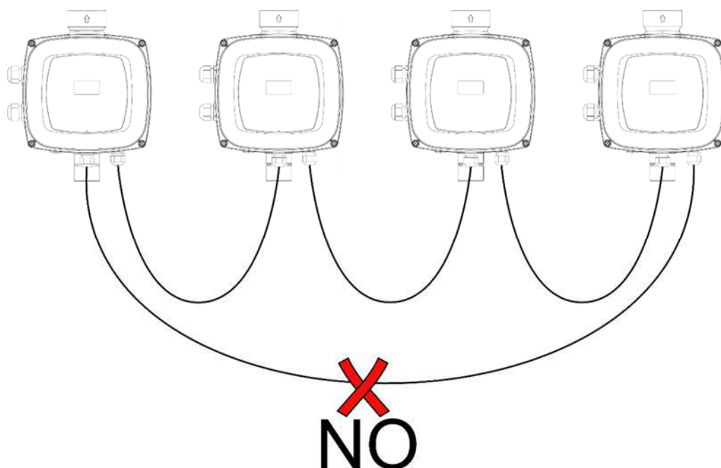
Rysunek 7: Nie wykonywać połączenia na pierścieniach
