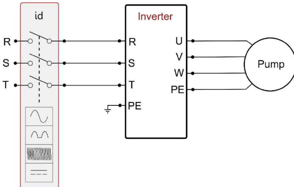
3b.: Ábra Installációs példa háromfázisos ellátás esetén
