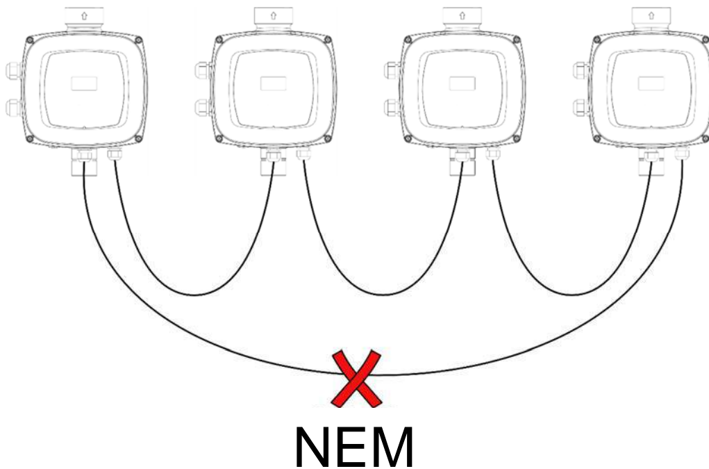
6. Ábra: Példa multi inverteres kommunikációs összekötésre 4 db.berendezéshez
