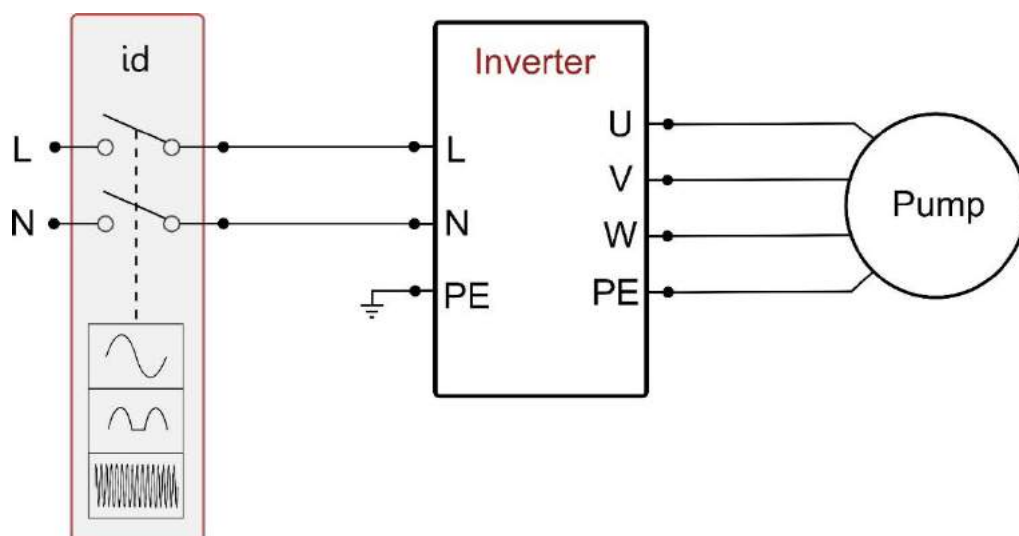
Figura 2a: Esempio di installazione con alimentazione monofase
