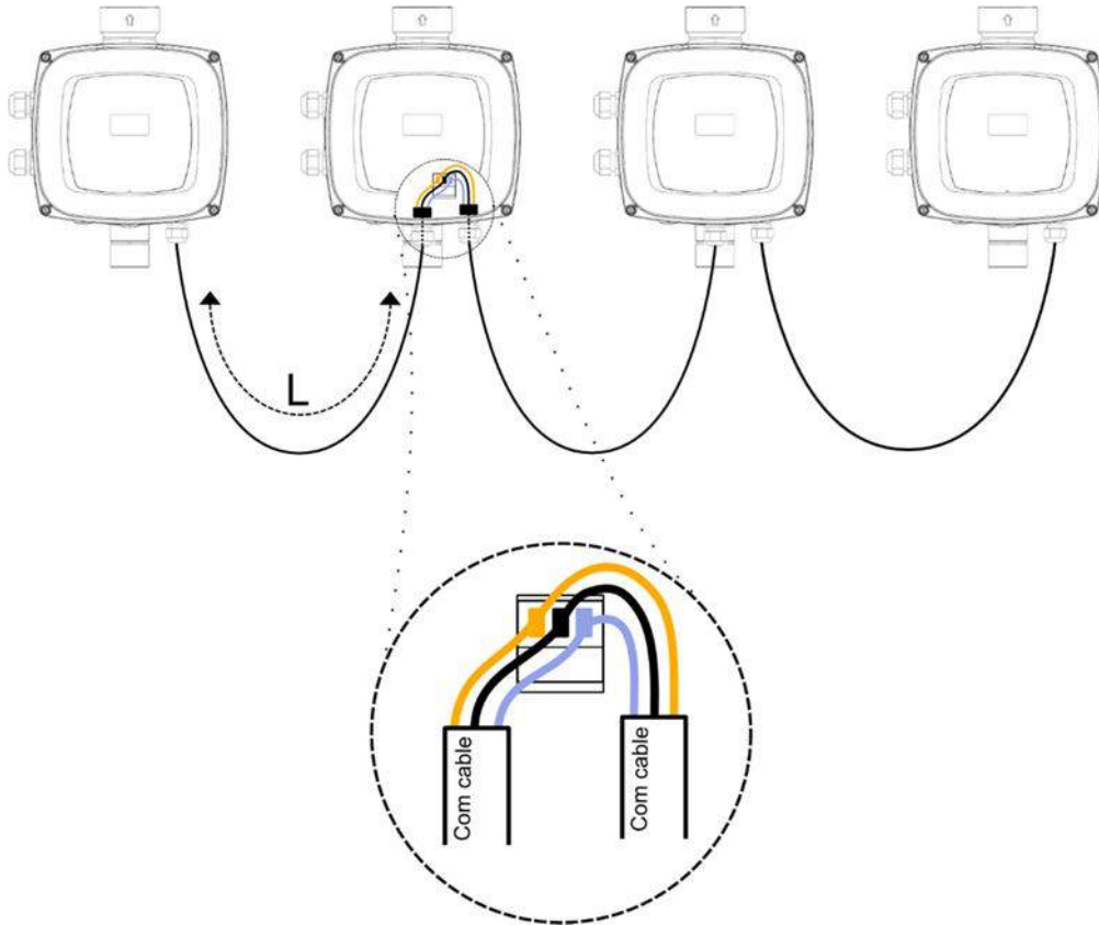
Kuva 6: Esimerkki 4 laitteen moni-invertterijärjestelmän yhteyskytkennästä
