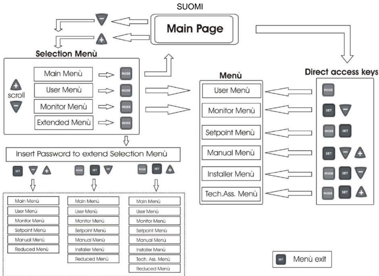
Kuva 13: Valikoiden avauskaavio
