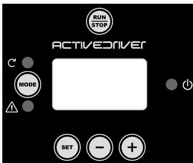
Fig. 11: Gränssnittets utseende
