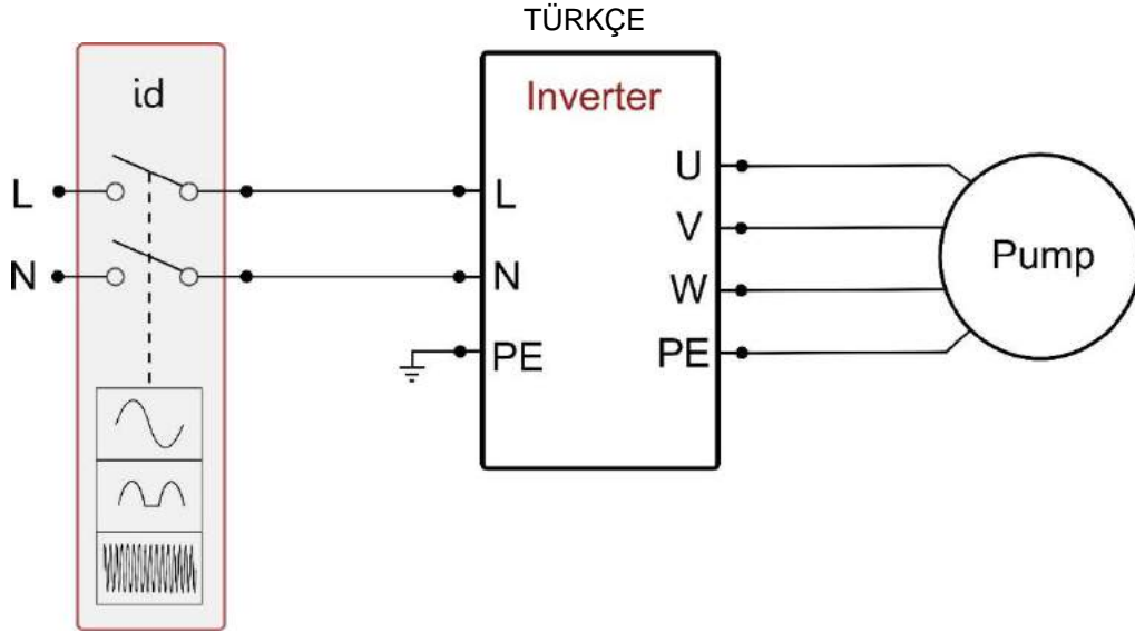
Şekil 2a: Monofaze besleme ile kurma örneğifofase
