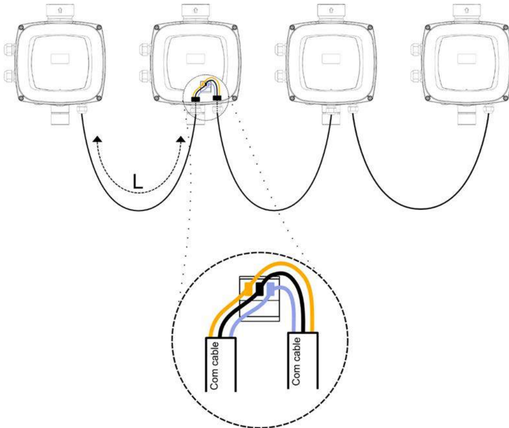
6. Ábra: Példa multi inverteres kommunikációs összekötésre 4 db.berendezéshez
