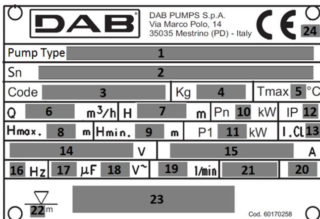
Fig. 3 Targhetta di identificazione
