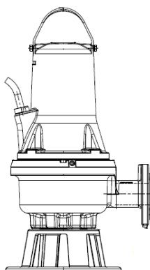
Obr. 7 Instalace ponorného čerpadla na podpěrný podstavec
