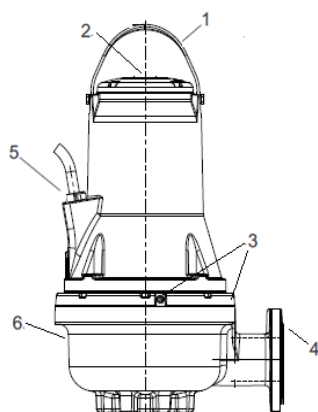
Obr. 1 Čerpadlo FK
