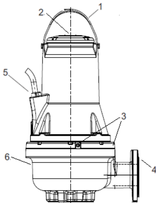
Kuva 1 FK -pumppu
