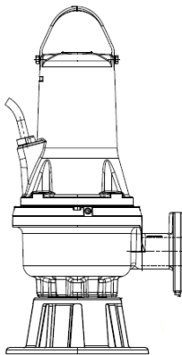
Abb. 7 Eingetauchte Installation auf Untergestell
