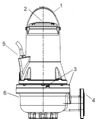
Fig. 1 Bomba FK
