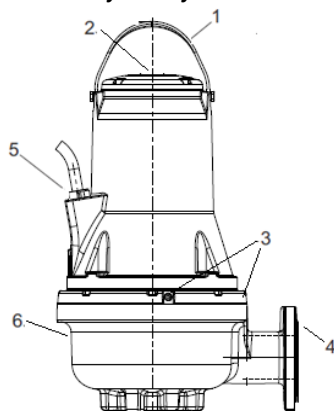
Obr. 1 Čerpadlo FK
