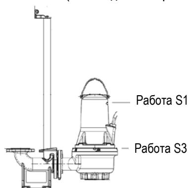
Рис. 2 Уровни остановки
