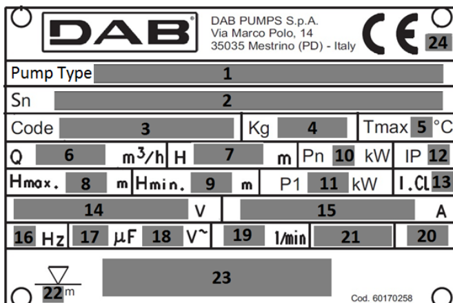
Slika 3 Natpisna pločica
