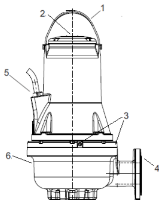
Fig. 1 Pompe FK
