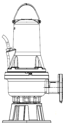
Slika 7 Uronjena instalacija na noseću bazu
