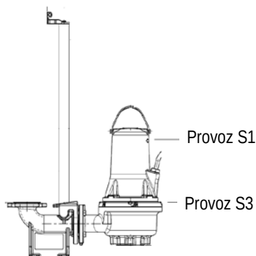
Obr. 2 Vypínací hladiny
