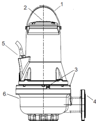
Joonis 1 Pump FK
