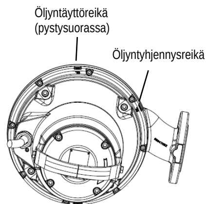
Kuva 11 Öljyn täyttöaukot
