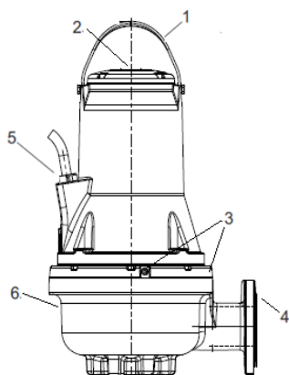
Slika 1 FK črpalka
