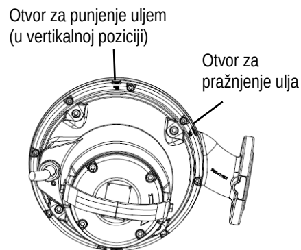
Slika 11 Punjenje uljem
