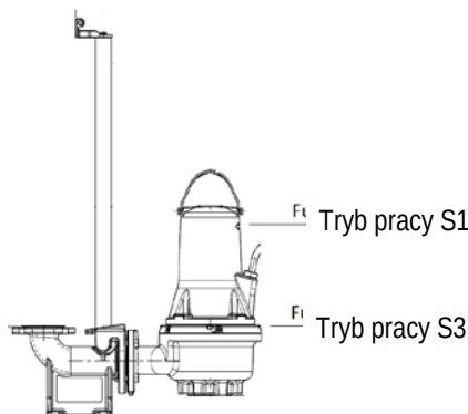
Rys. 2 Poziomy wyłączania
