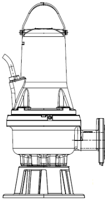
Joonis 7 Märgpaigaldus tugialusele
