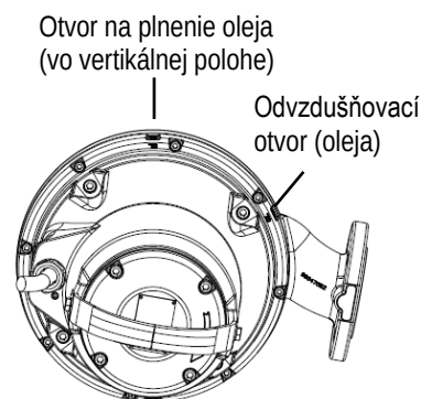
Obr. 11 Plniace otvory na olej
