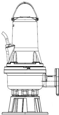
Fig. 7 Instalación sumergida sobre base de soporte
