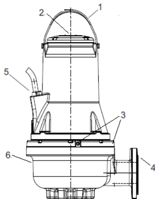
Slika 1 FK crpka
