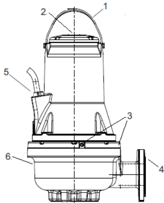
Мал. 1 Насос FK
