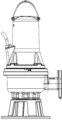
Şekil 7 Destek tabanı üzerine daldırılmış kurulum tipi
