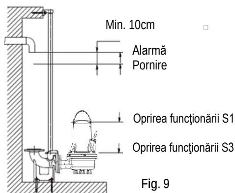
Fig. 9 Nivelurile de pornire și oprire Asigurați-vă că volumul efectiv al lichidului din rezervor nu scade atât încât numărul pornirilor pe oră să depășească numărul maxim permis.
