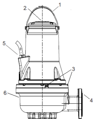
Fig. 1 Pompa FK
