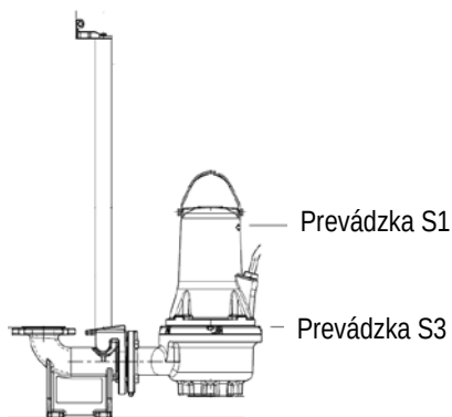
Obr. 2 Vypínacie hladiny
