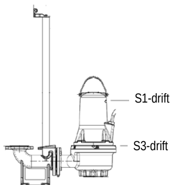
Fig. 2 Stoppnivåer
