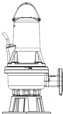
Slika 7 Uronjena instalacija na potpurnu osnovu
