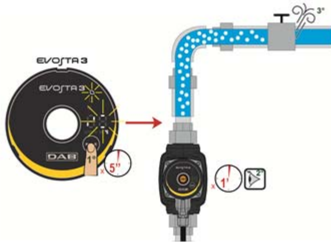
Abb. 9: Automatische Pumpenentlüftung
