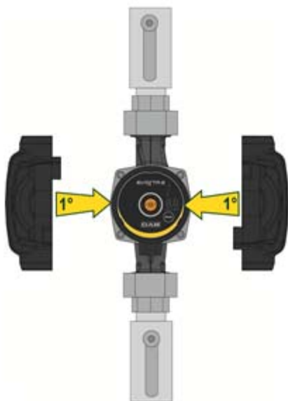
Figura 5: Aislamiento del cuerpo de la bomba
