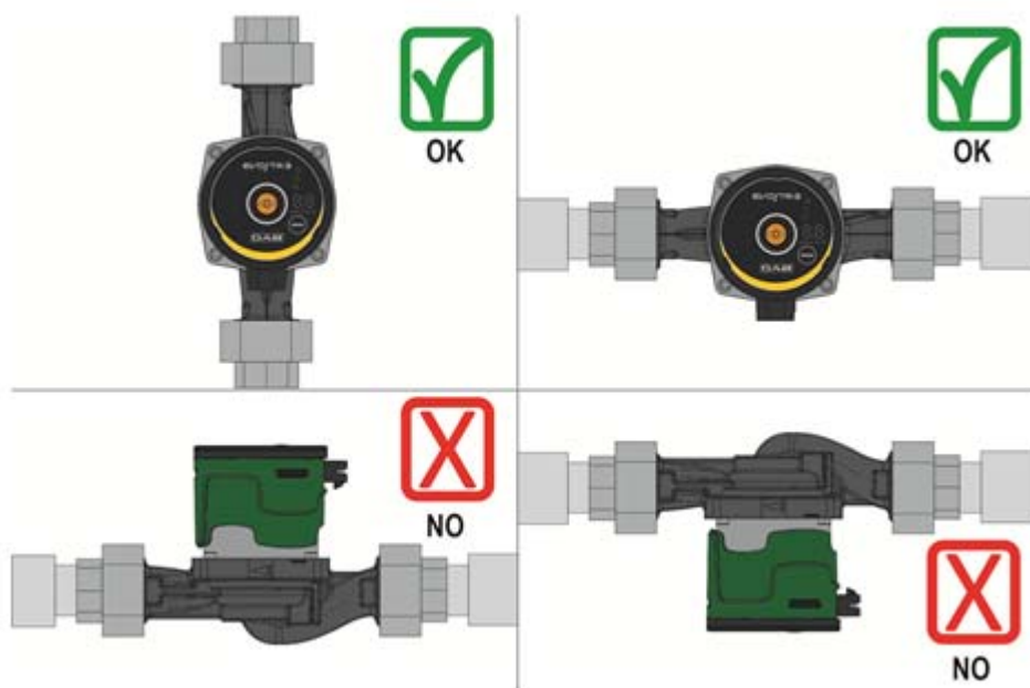
Εικόνα 3: Θέση συναρμολόγησης
