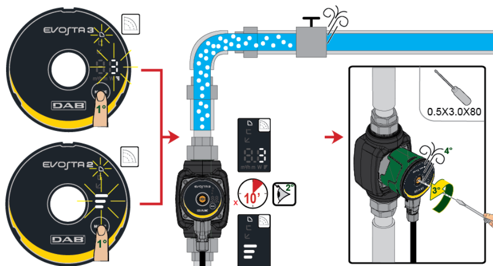
Slika 8: Odzračitev črpalke
