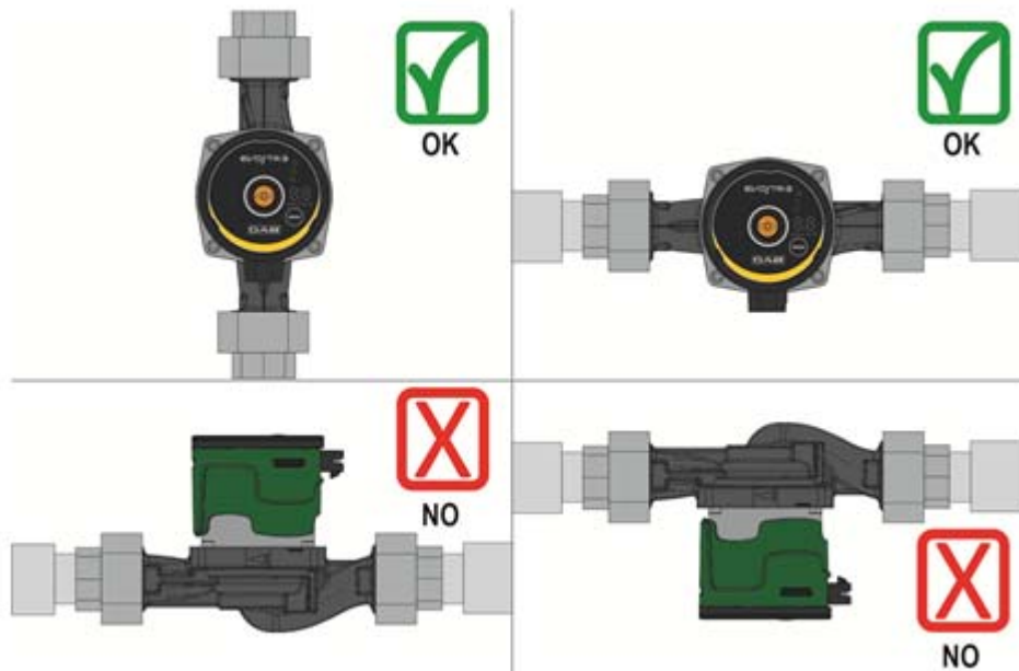
Kuva 3: Asennusasento
