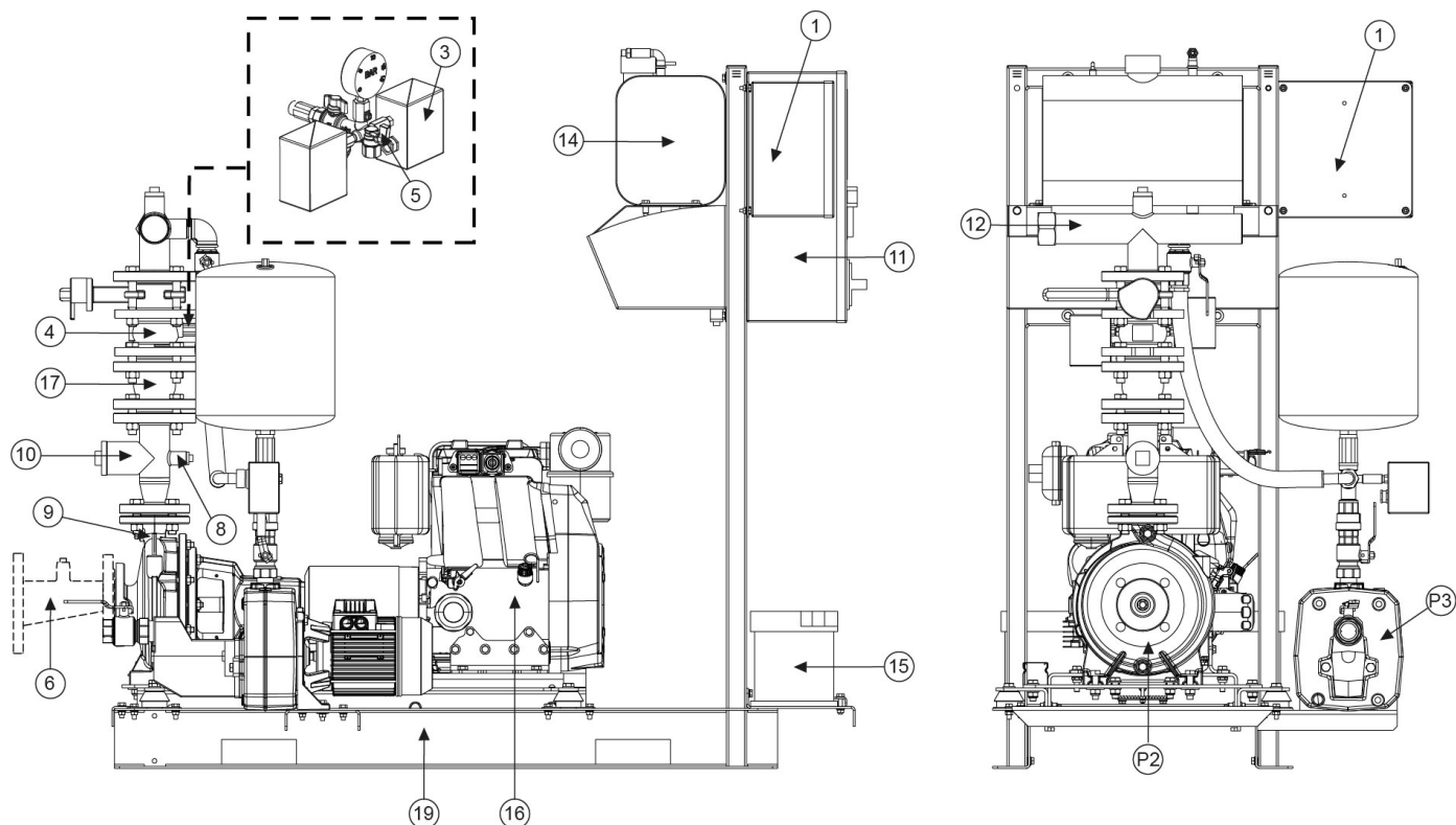
Головний електронасос
