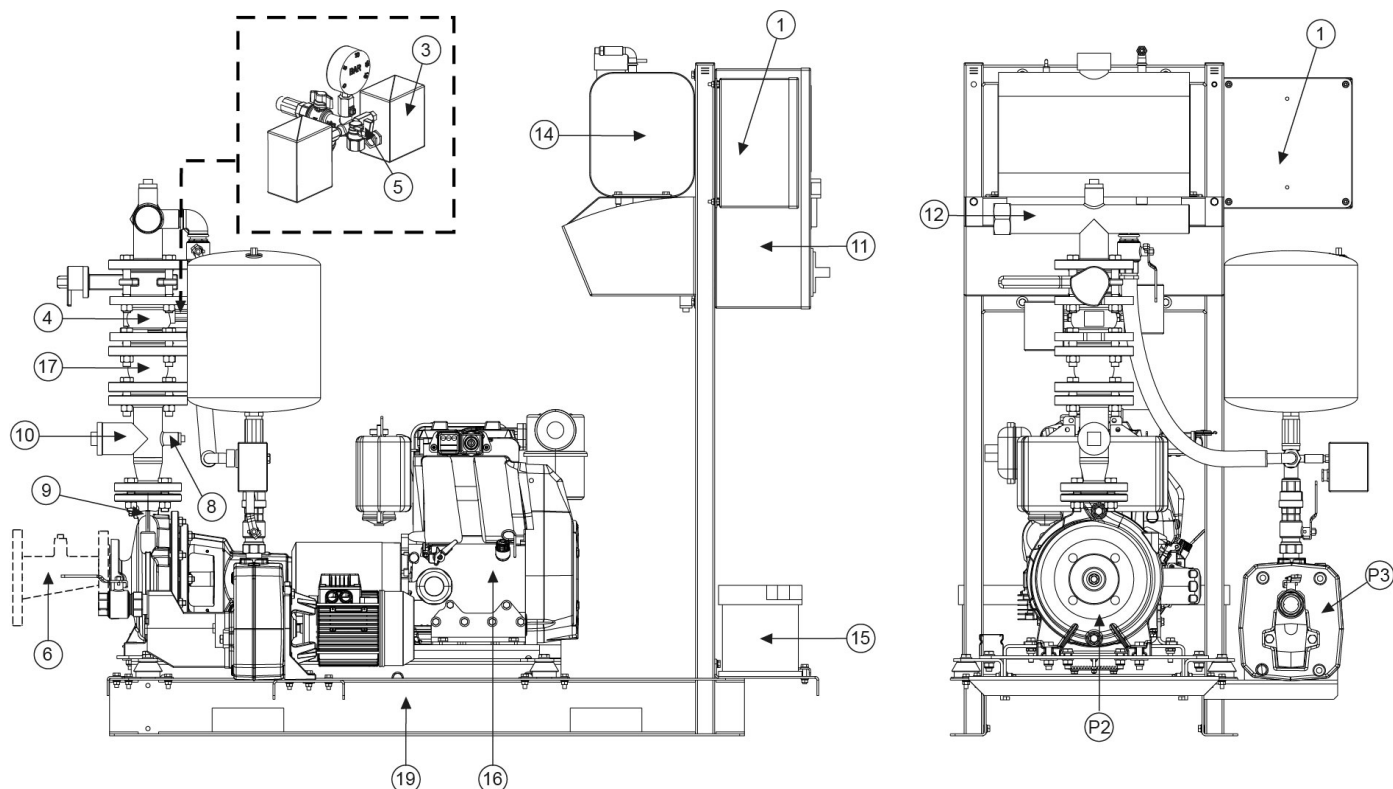
Główna pompa
