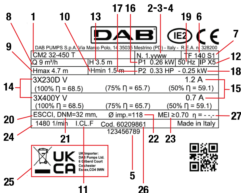
Fig.1 Etiqueta
