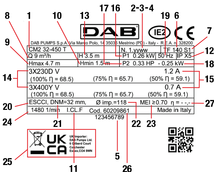
1 pav. Plokštelė
