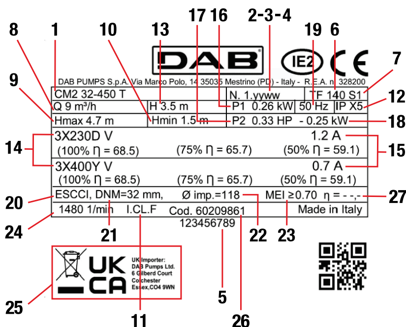
Fig.1 Märkplåt
