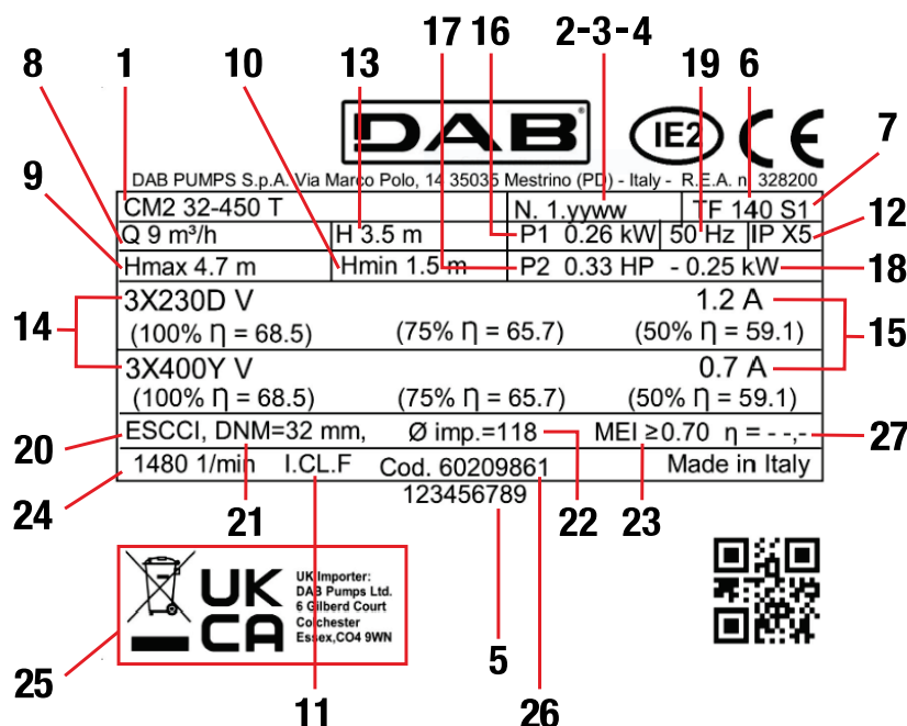
Abb. 1 Typenschild
