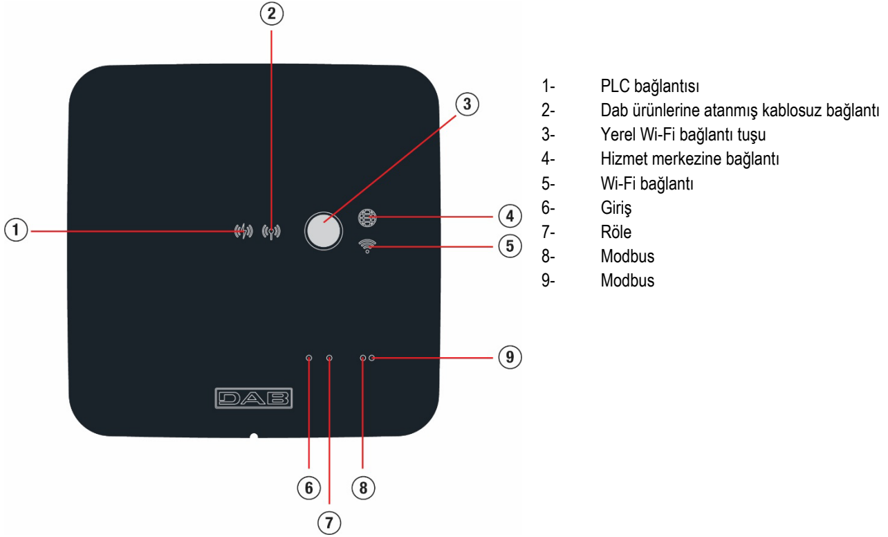
Göstergelerin Anlamları
