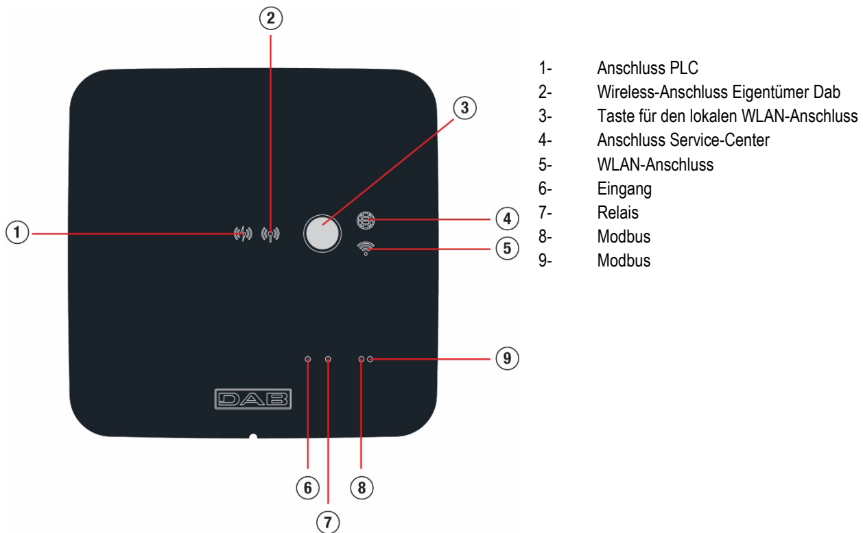
Bedeutung Anzeiger
