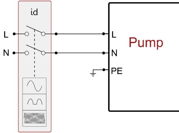
Montaj Örneği
