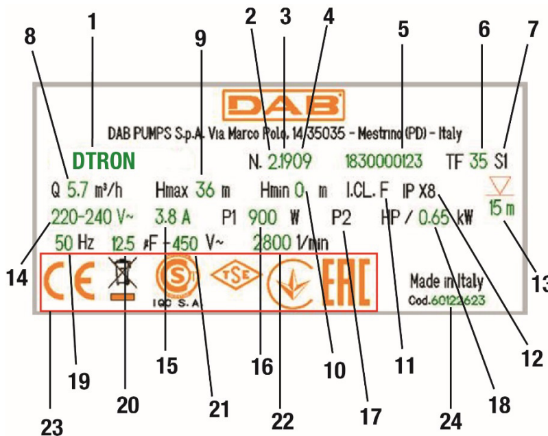
Kennzeichen
