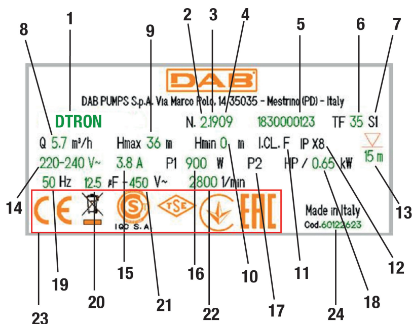
Eticheta tehnică
