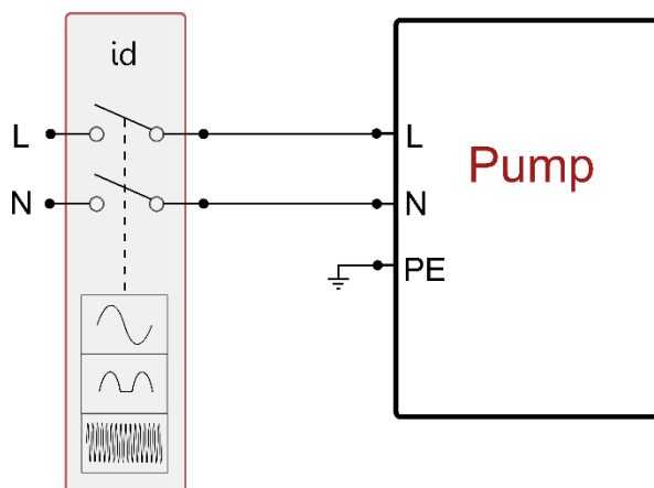
Esimerkki asennuksesta
