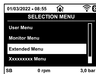
Figura 13.2: Meniu derulant (3) (4)
