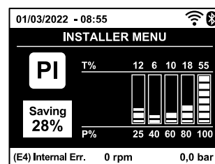
Фиг 17.2: Хистограма (3) (4)
