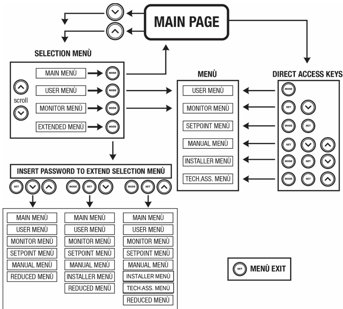
Kuva 14 Valikoiden avauskaavio
