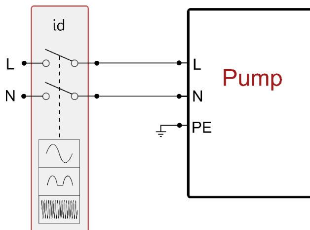
Obr. 10 Příklad instalace
