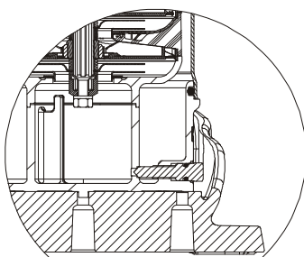
ЗЛИВНИЙ ОТВІР
