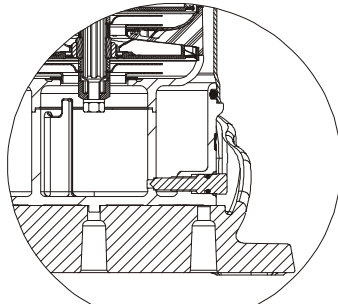
غطاء التفريغ
