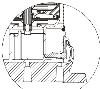
ΤΑΠΑ ΕΚΚΕΝΩΣΗΣ
