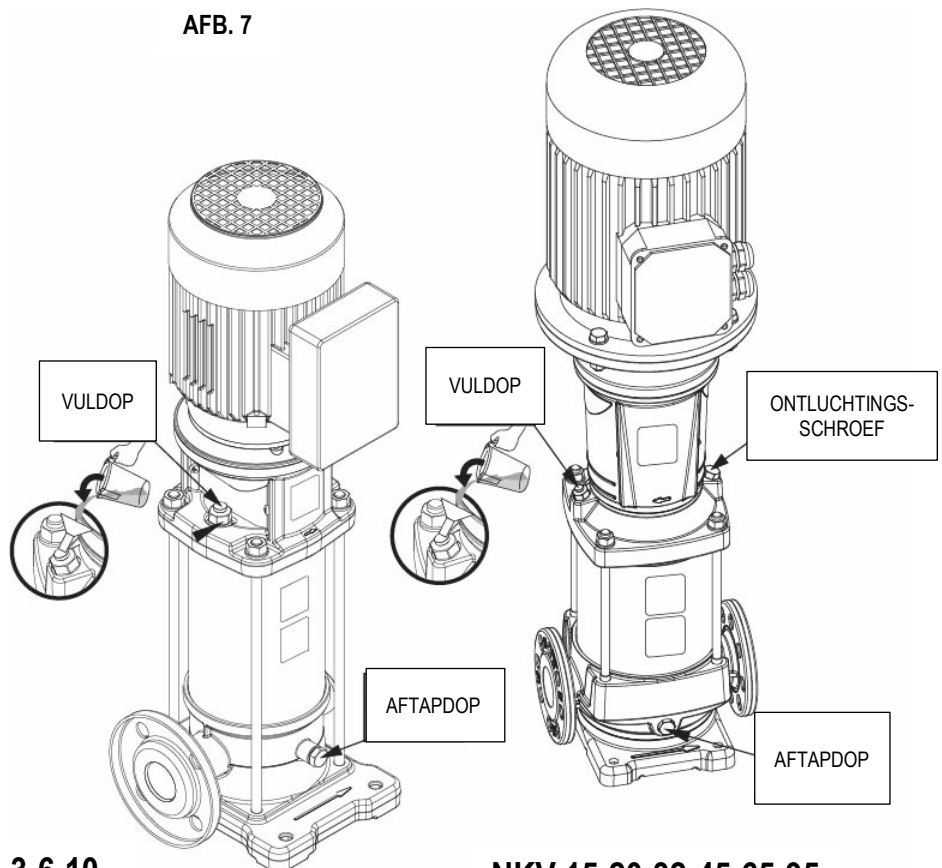
NKV 15-20-32-45-65-95
