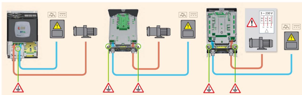
Figure 6: Connexions électriques
