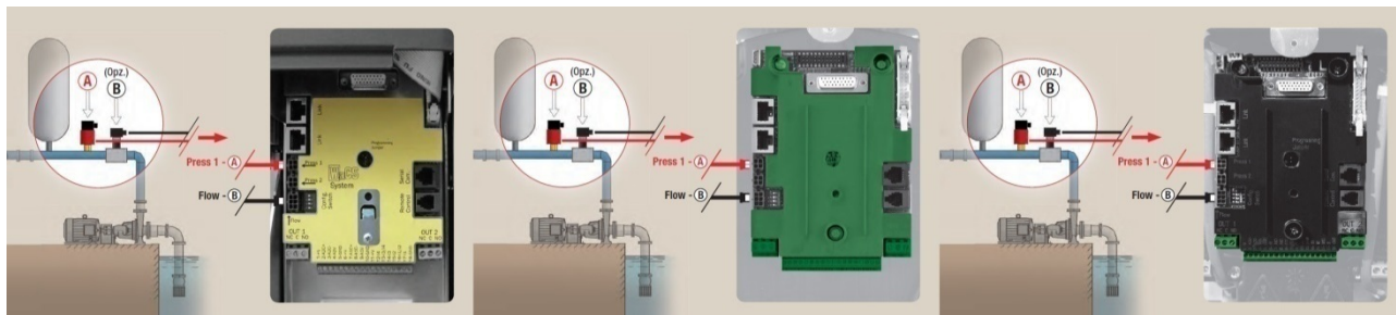
Obrázek 9: Připojení snímačů
