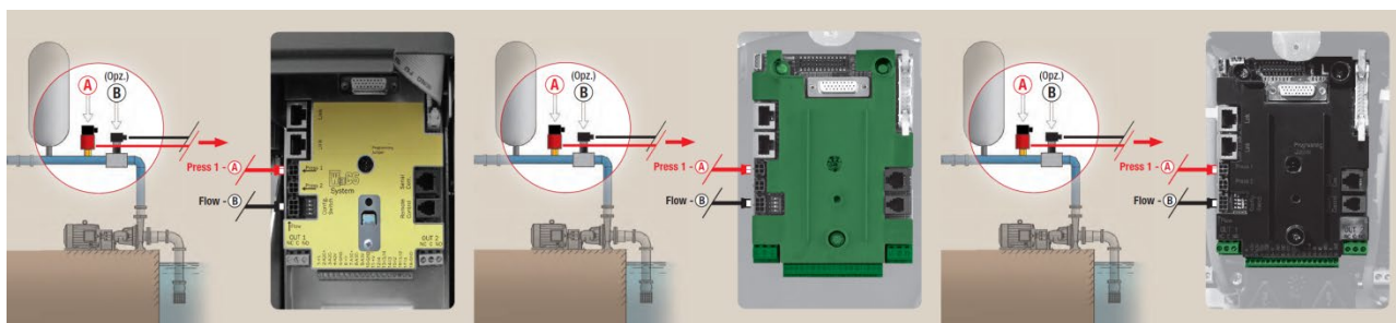
Рисунок 9: З'єднання датчиків
