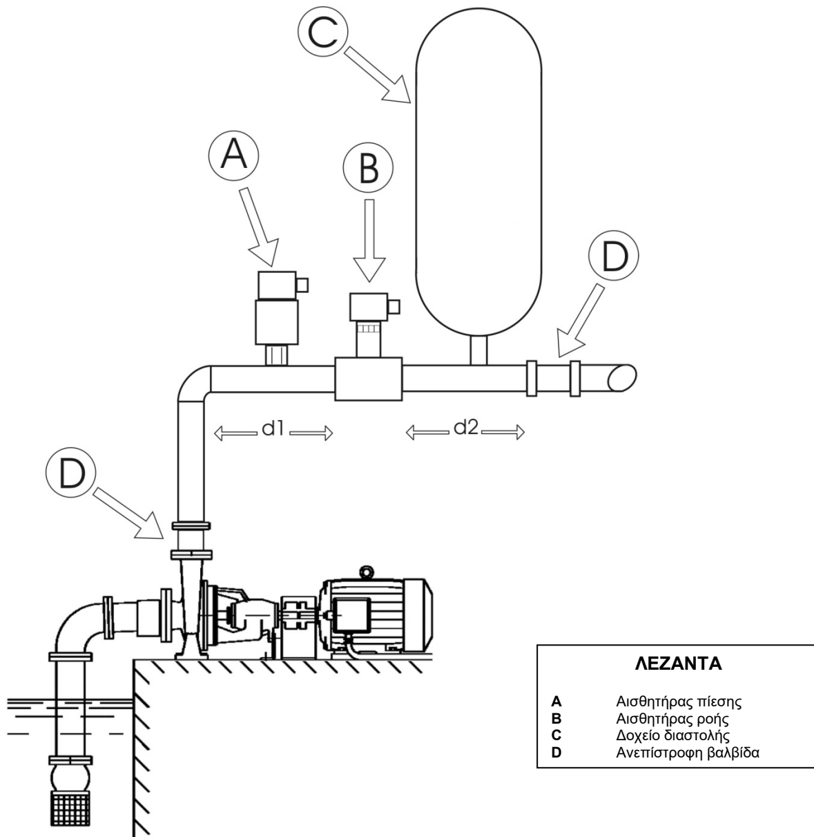
Σχήμα 8: Υδραυλική εγκατάσταση
