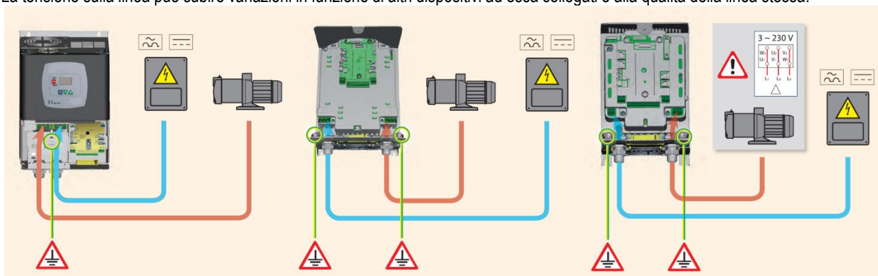
Figura 6: Connessioni elettriche
