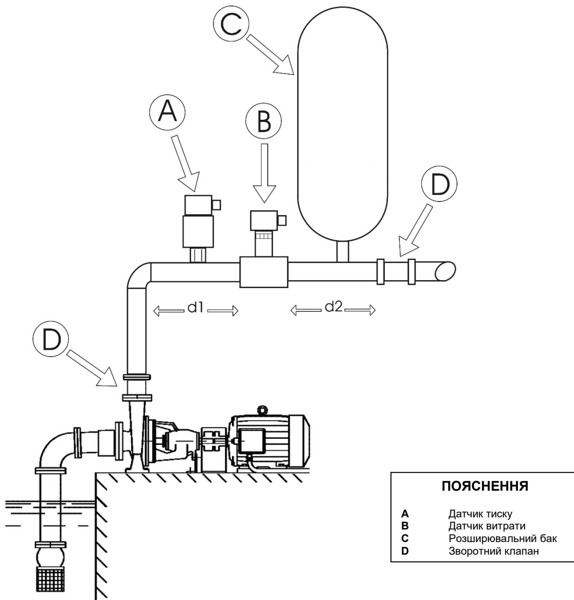
Рисунок 8: Гідравлічний монтаж
