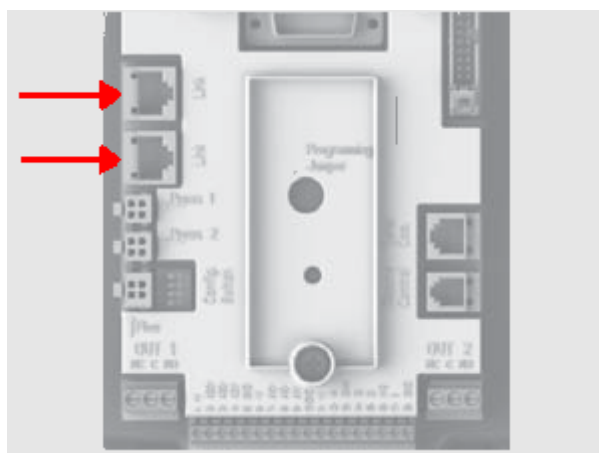
Figura 18: Conexión Link
