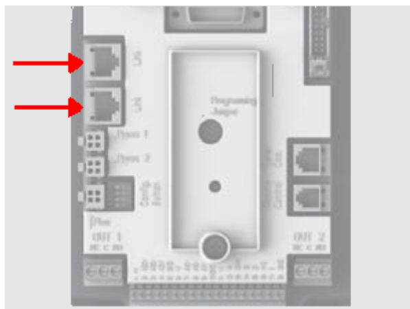
Abbildung 18: Link-Anschluss 214
