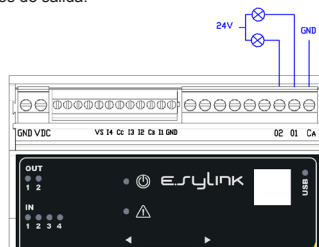
Figura 3: Ejemplo de conexión salidas
