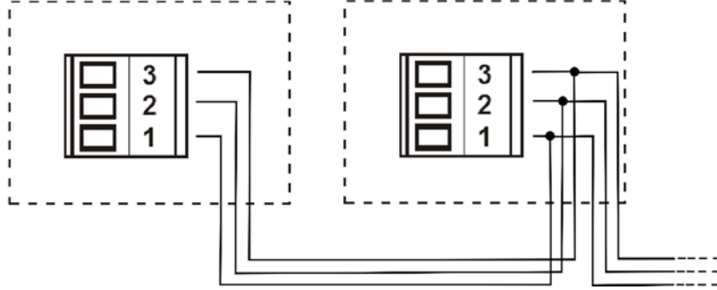
Şekil 4: Multi invertör haberleşme bağlantısı
