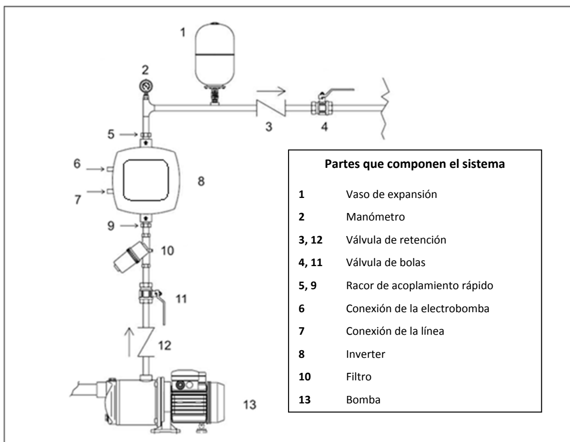
Figura 1: Instalación hidráulica
