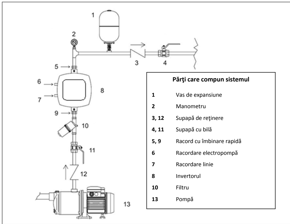
Figura 1: Instalație hidraulică
