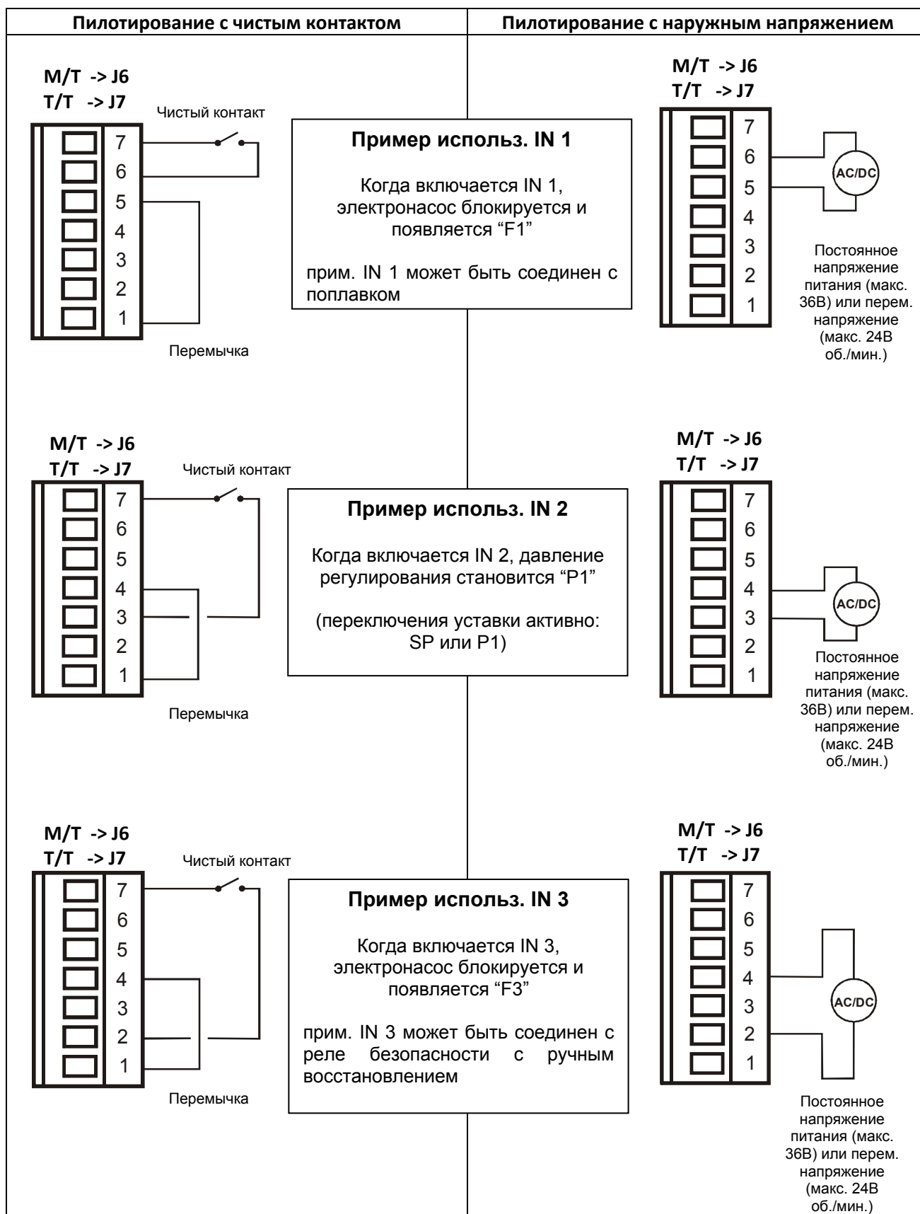
Рисунок 2: Соединение входов
