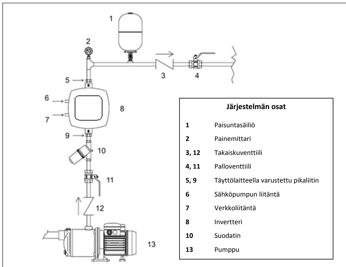
Kuva 1: Vesijärjestelmä
