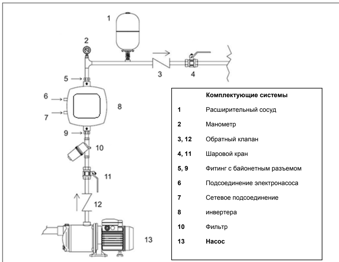
Рисунок 1: Гидравлическая установка
