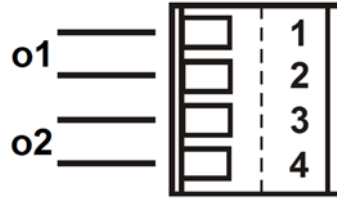
Şekil 3: Çıkışların bağlantısı
