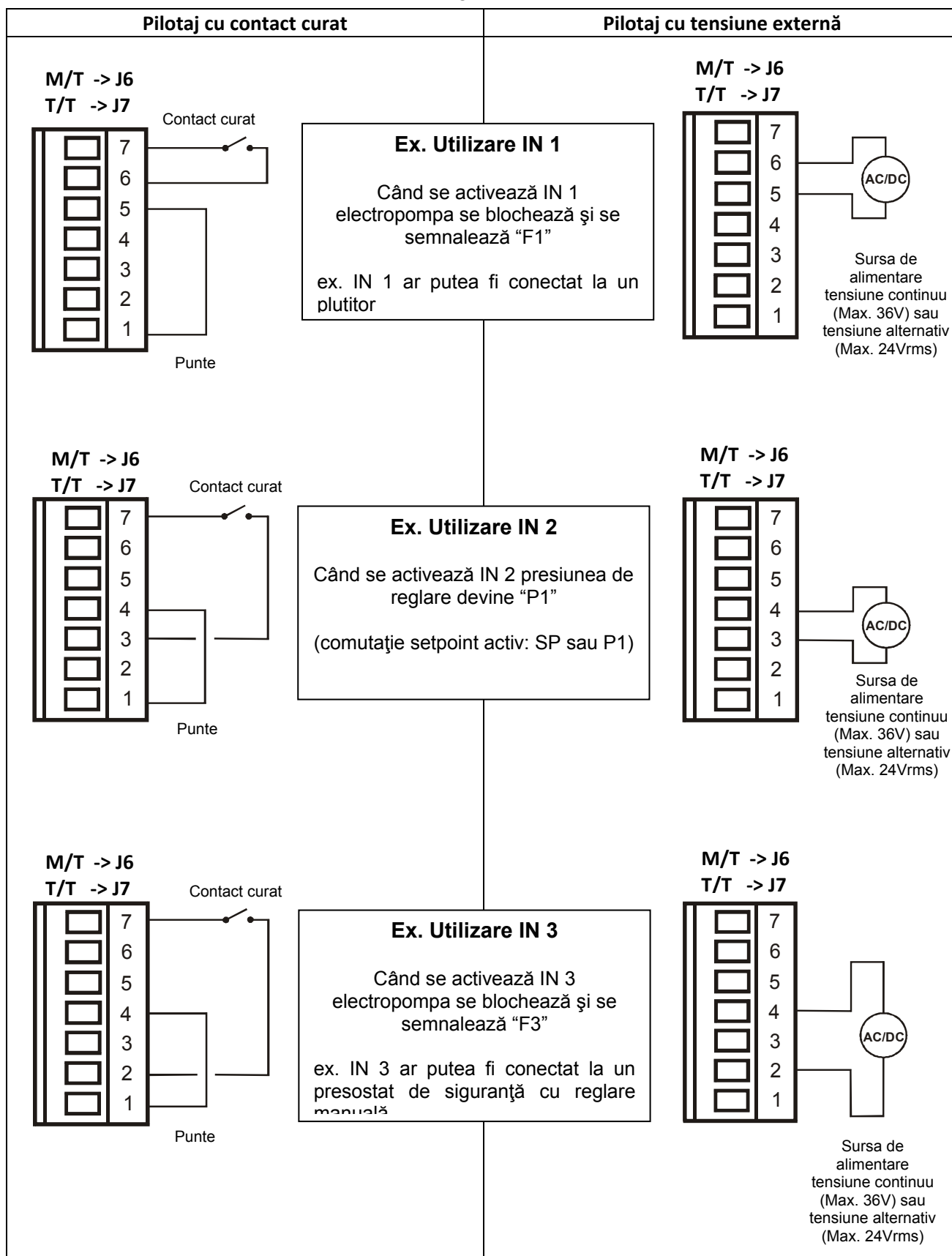
Figura 2: Conexiune intrări
