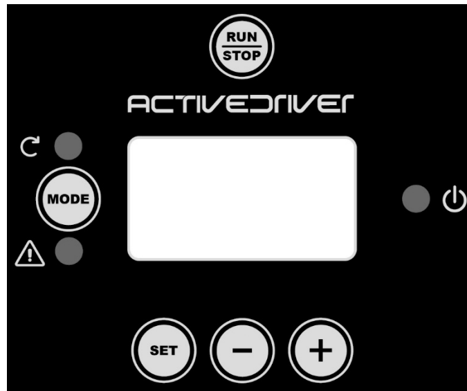
Kuva 6: Käyttöliittymän ulkomuoto
