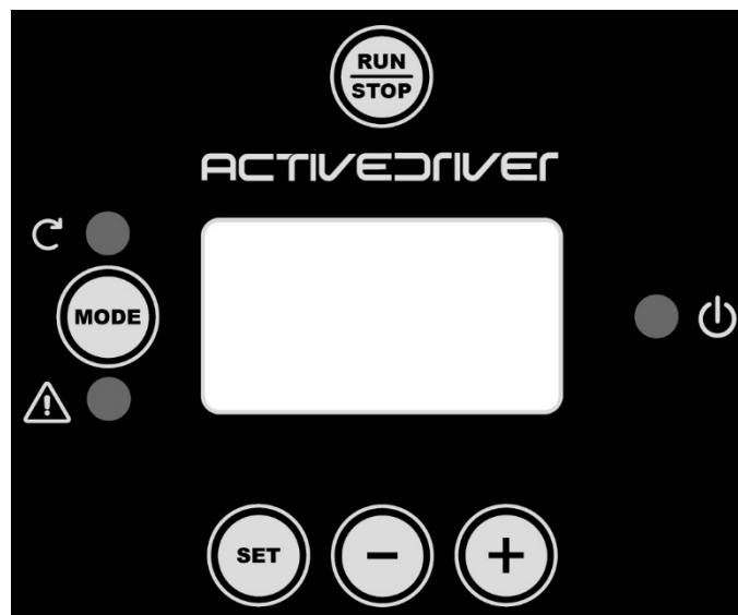
Fig. 6: Gränssnittets utseende
