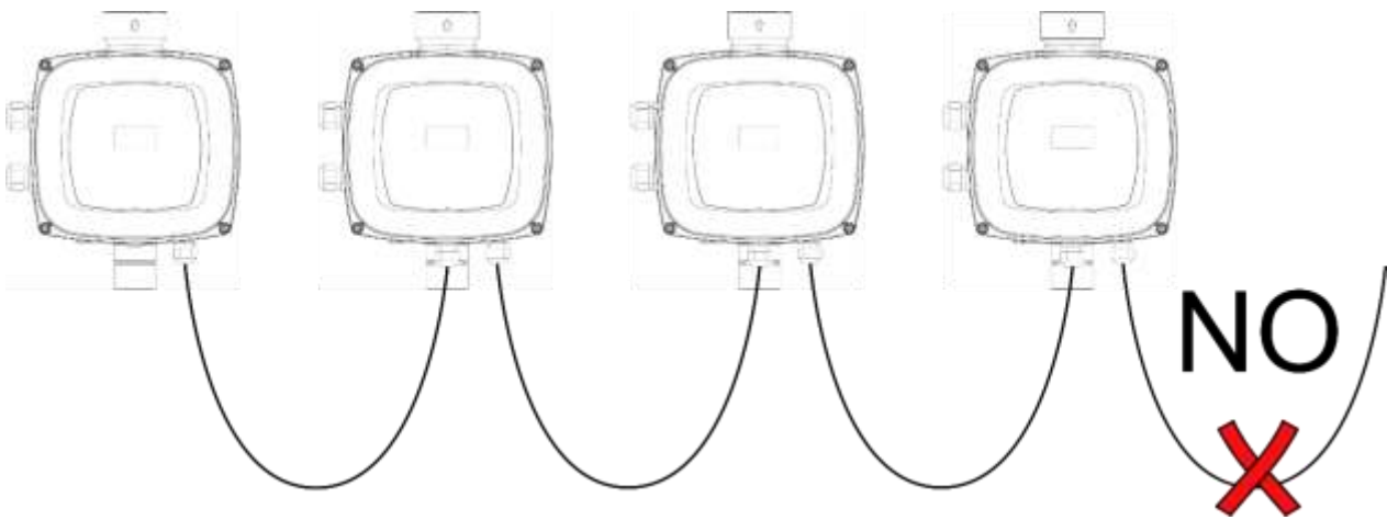
Figure 9: Ne pas laisser les câbles branchés à une seule extrémité
