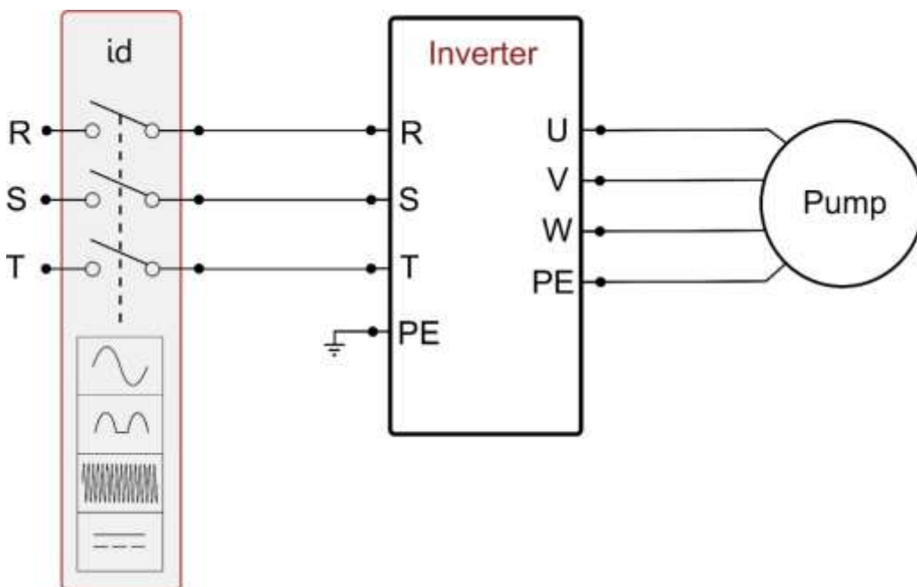
Kuva 3b: Asennusesimerkki kolmivaiheisella virtalähteellä
