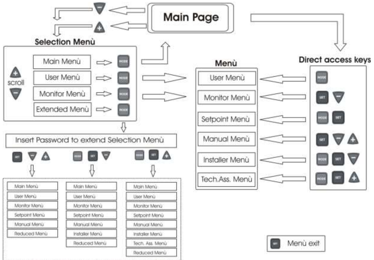
13. Ábra: A menükhöz való belépési lehetőségek sémája
