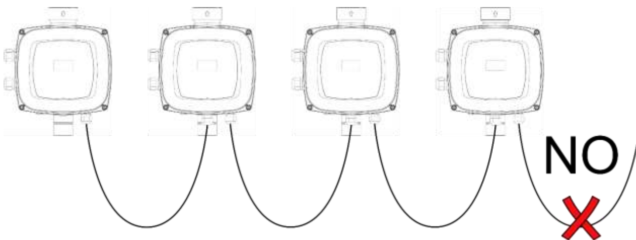
Fig. 9: Lämna inte kablar anslutna i bara ena änden
