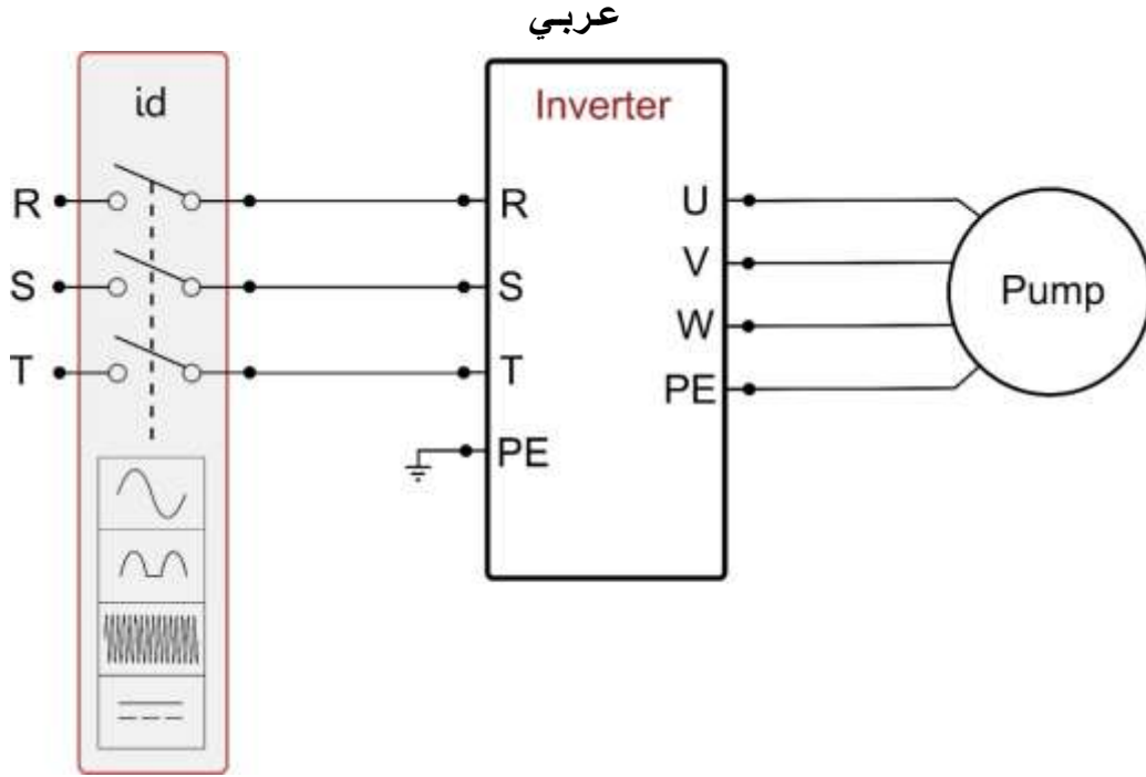
رسم رقم b2: مثال تركيب مع تموين ثلاثي الطور
