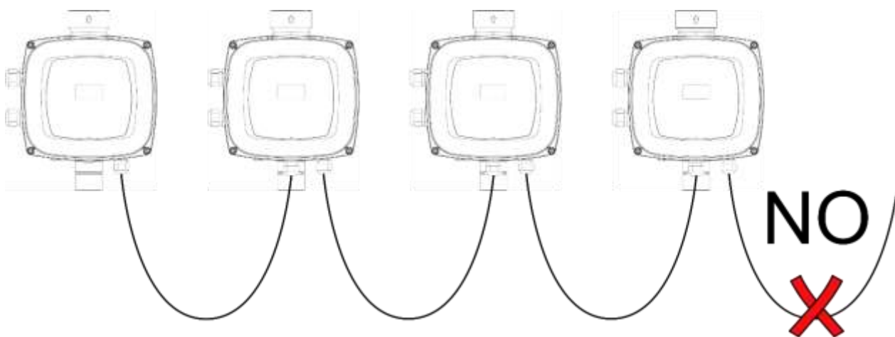
Kuva 9: Älä jätä johtoja kytketyiksi ainoastaan yhdestä päästä
