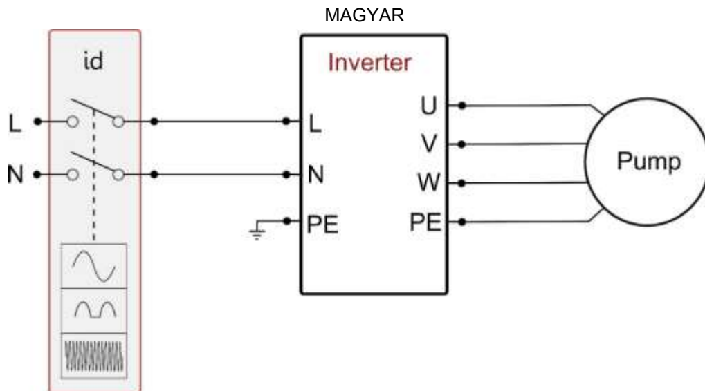
2a.: Ábra Installációs példa monofázisos ellátás esetén
