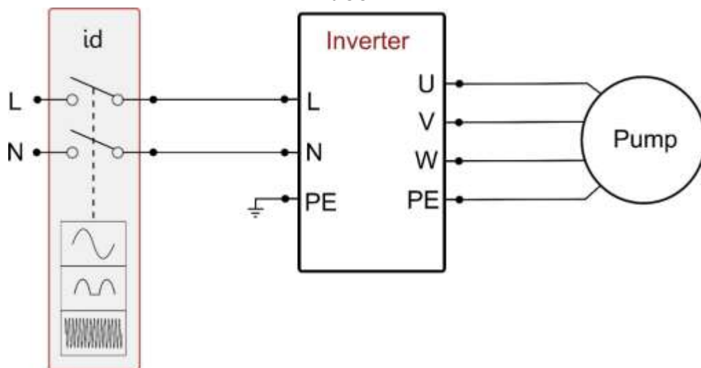
Рисунок 2а: Пример установки при однофазном питании
