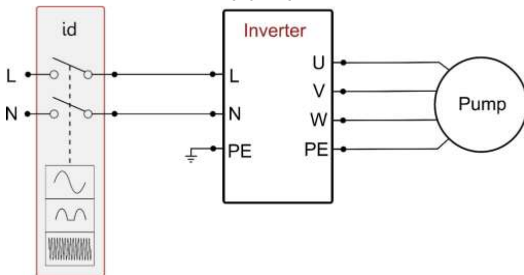
Obrázok 2a: Príklad inštalácie s jednofázovým napájaním
