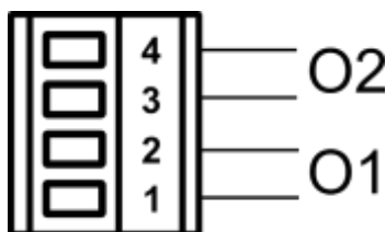
Obrázok 5: Pripojenie výstupov
