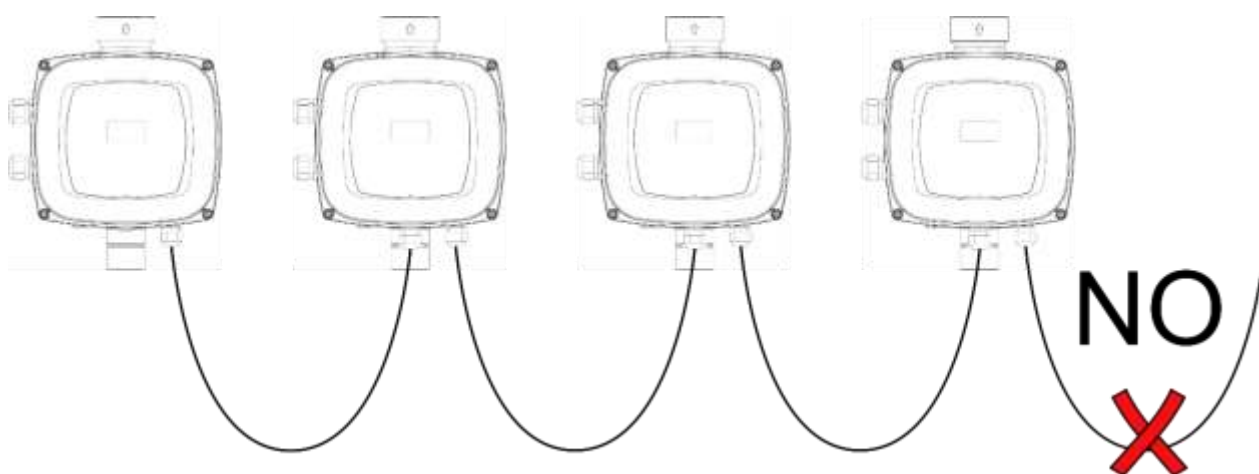
Rysunek 9: Nie pozostawiać kabli połączonych tylko na jednym końcu
