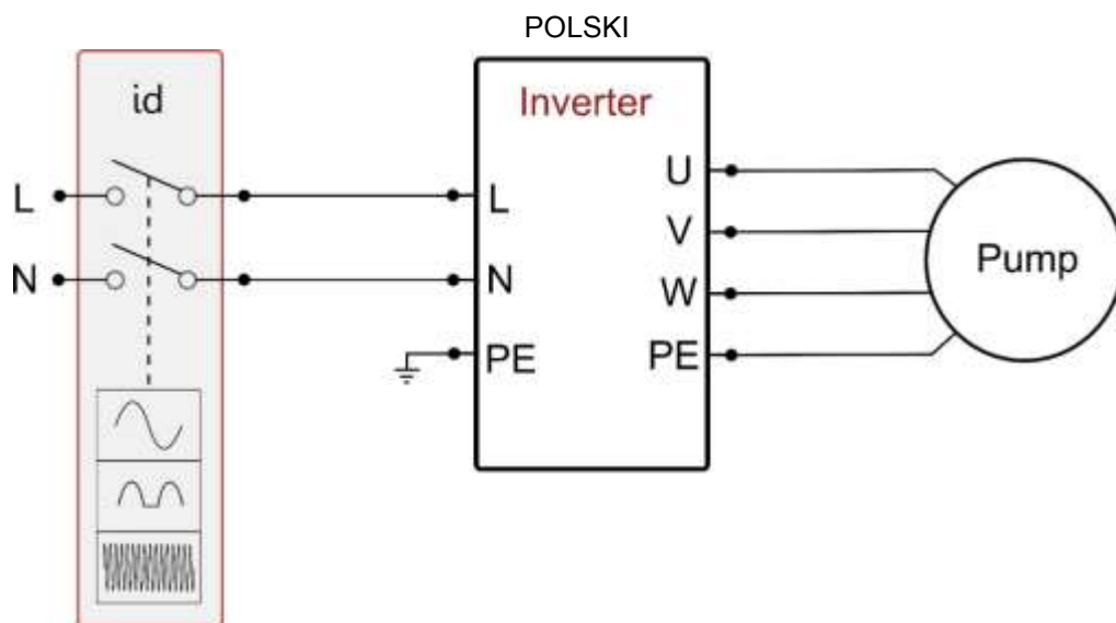
Rysunek 2a: Przykład zainstalowania z zasilaniem jednofazowym
