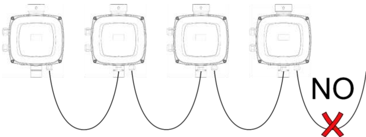
Σχήμα 9: Μην αφήνετε καλώδια συνδεδεμένα μόνο στο ένα άκρο
