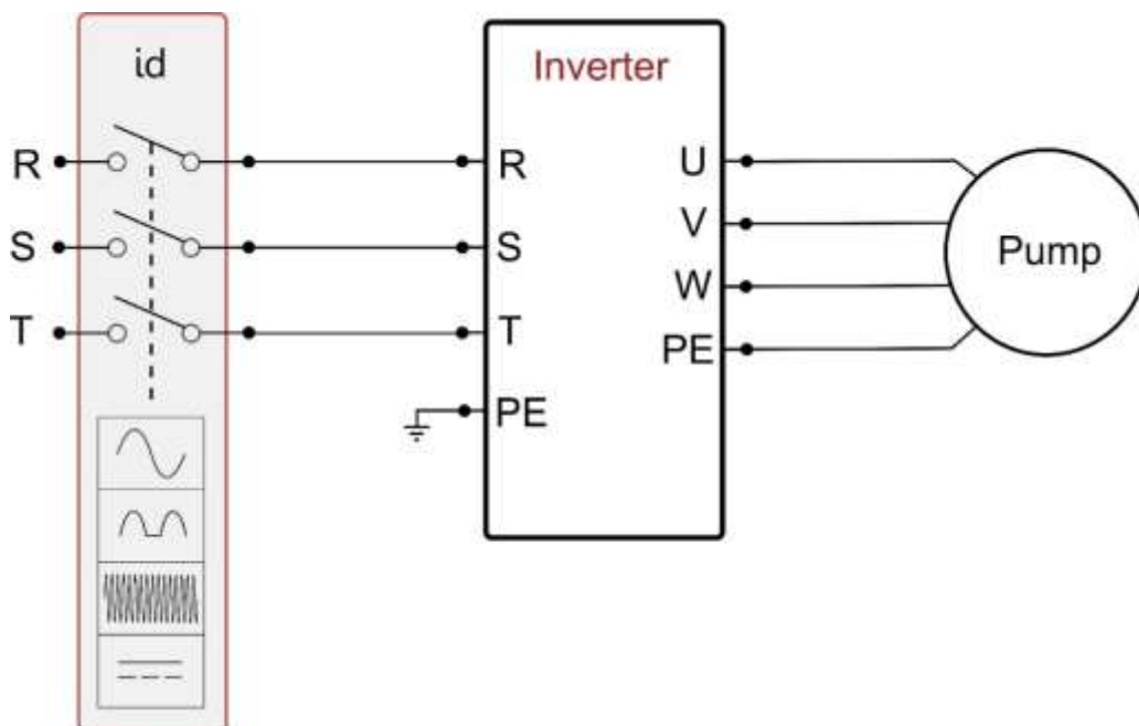
Рисунок 3b: Пример установки при трехфазном питании
