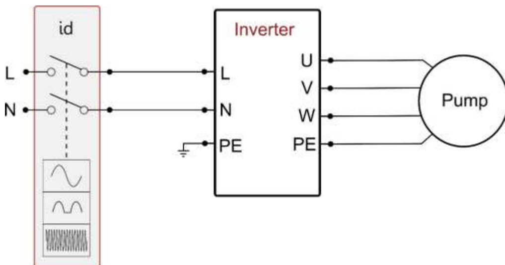
Kuva 2a: Asennusesimerkki yksivaiheisella virtalähteellä
