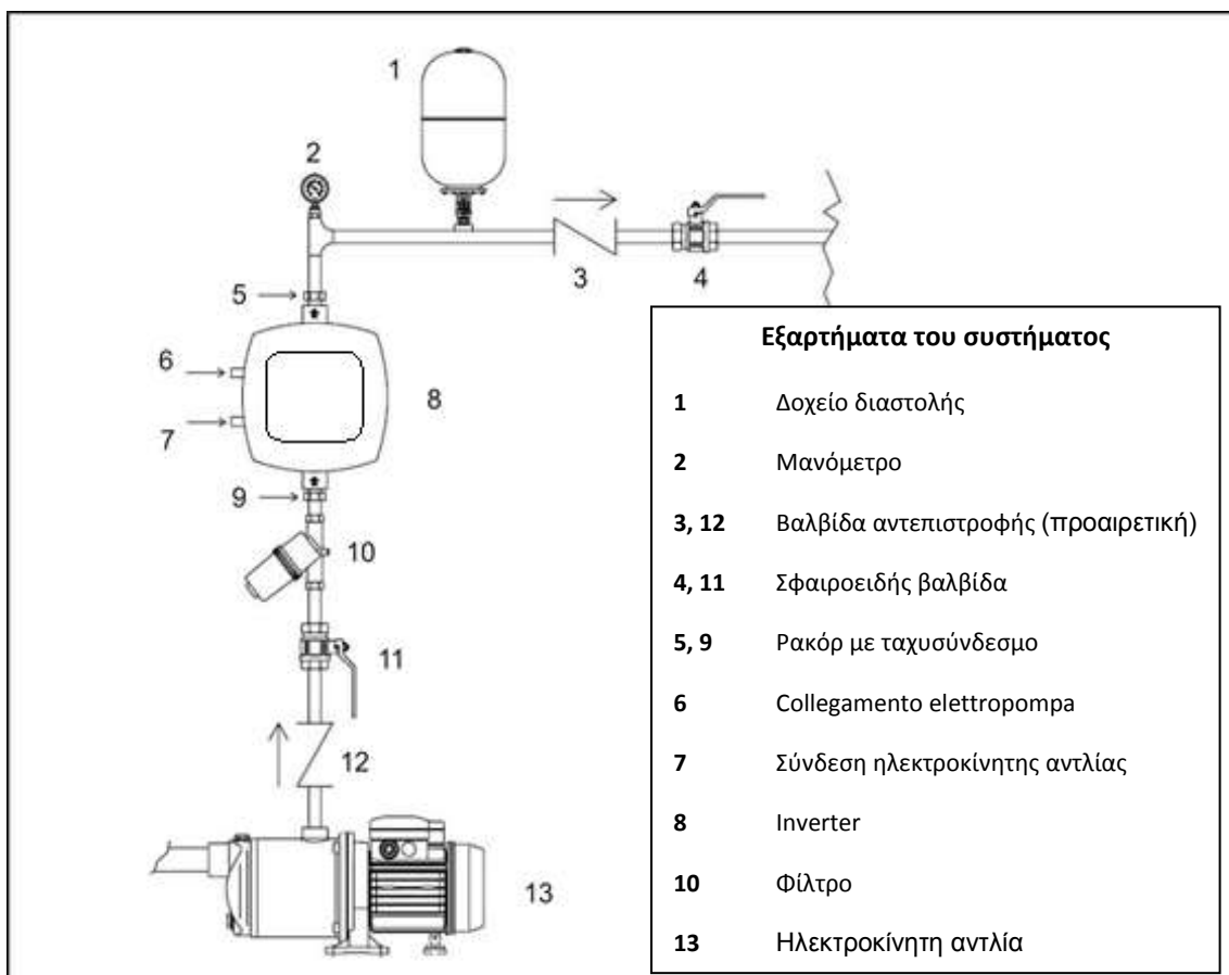
Σχήμα 1: Υδραυλική εγκατάσταση
