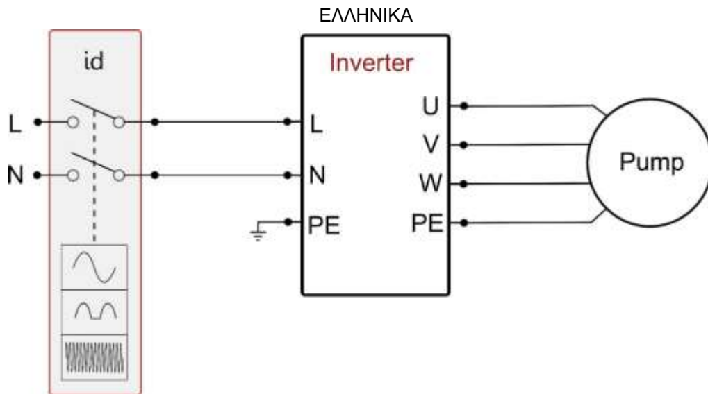
Σχήμα 2a: Παράδειγμα εγκατάστασης με μονοφασική τροφοδοσία
