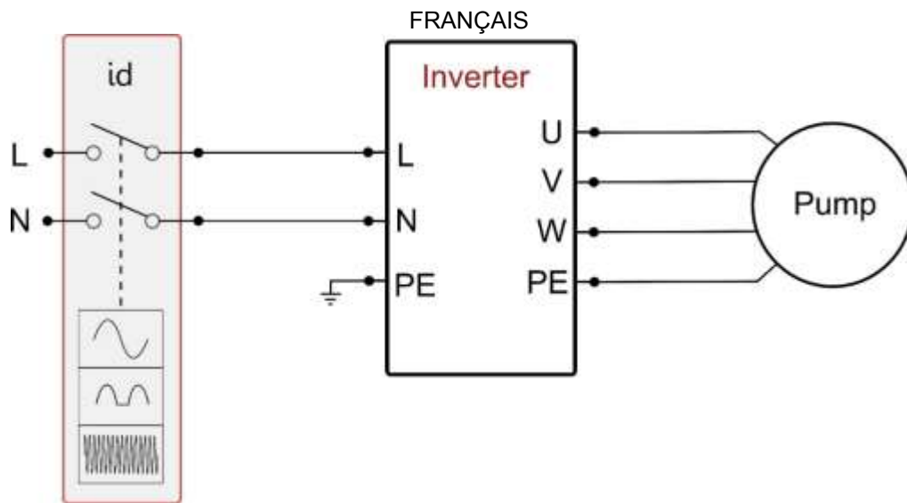
Figure 2a: Exemple d'installation avec alimentation monophasée
