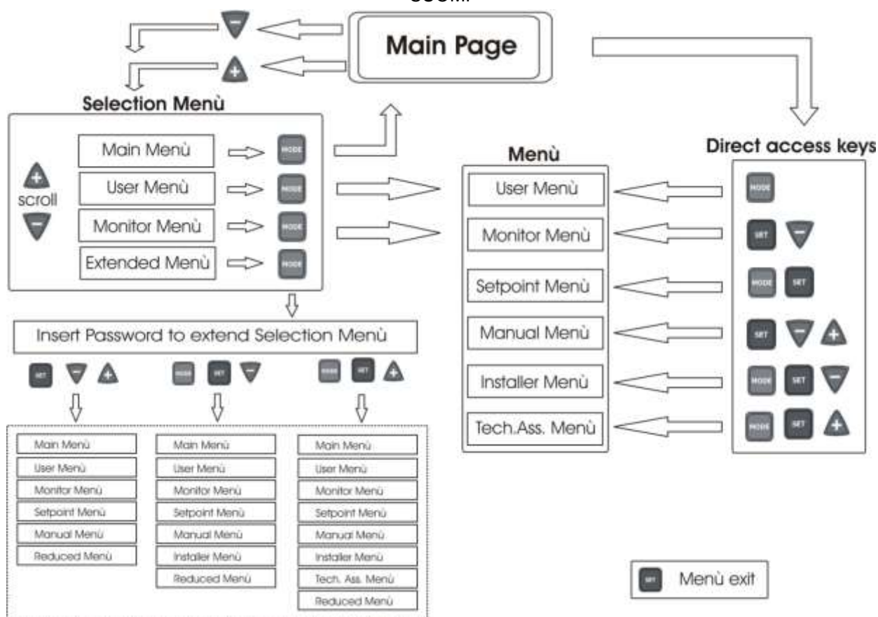
Kuva 13: Valikoiden avauskaavio
