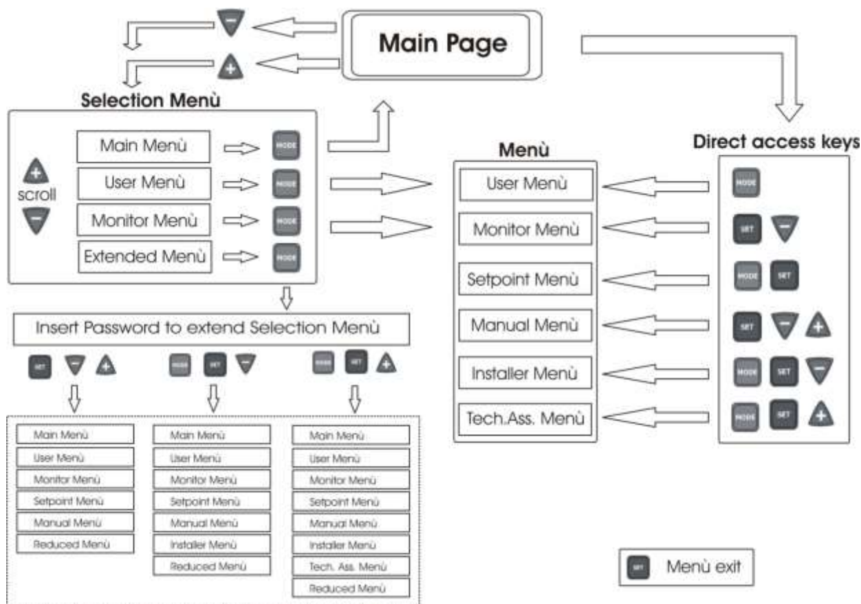
Σχήμα 13: Σχηματική αναπαράσταση των δυνατών προσβάσεων στα μενού
