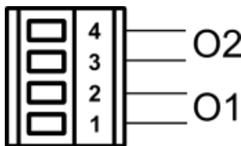
Abbildung 5: Anschluss der Ausgänge
