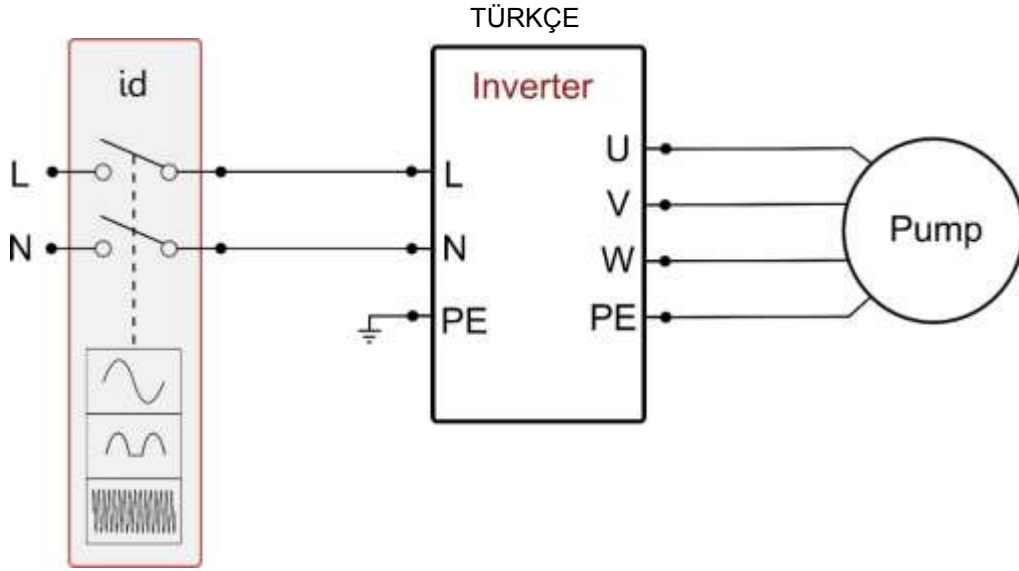
Şekil 2a: Monofaze besleme ile kurma örneğinofase
