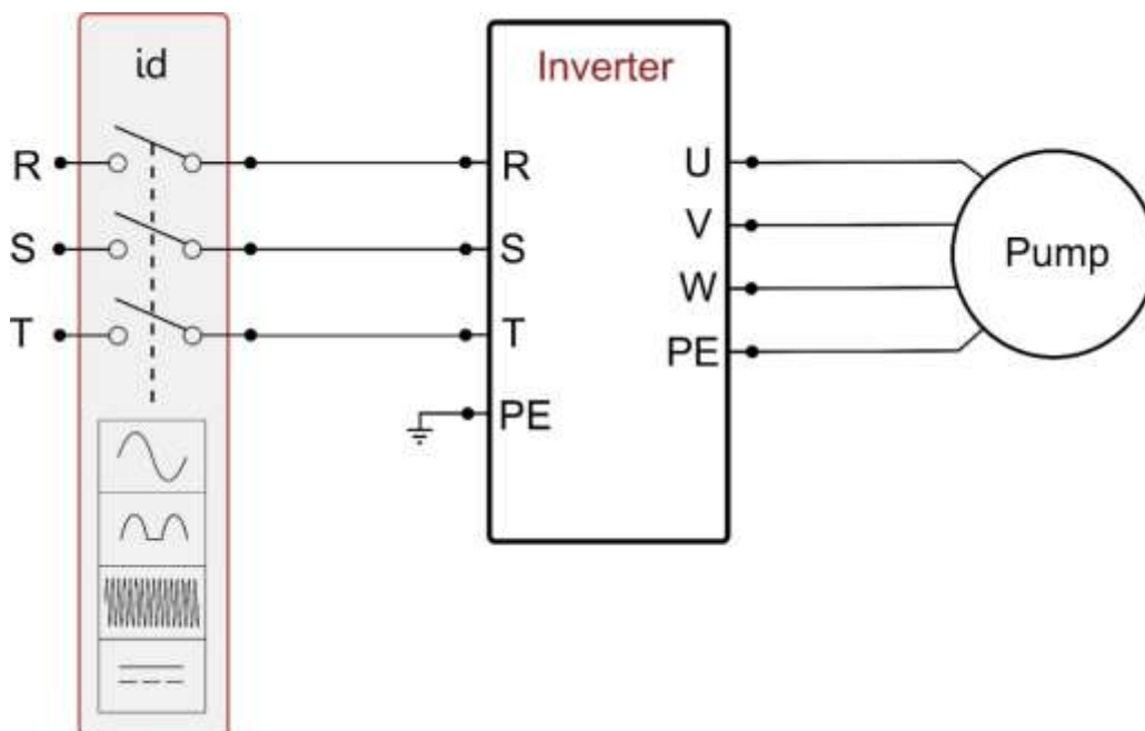
Σχήμα 3b: Παράδειγμα εγκατάστασης με τριφασική τροφοδοσία
