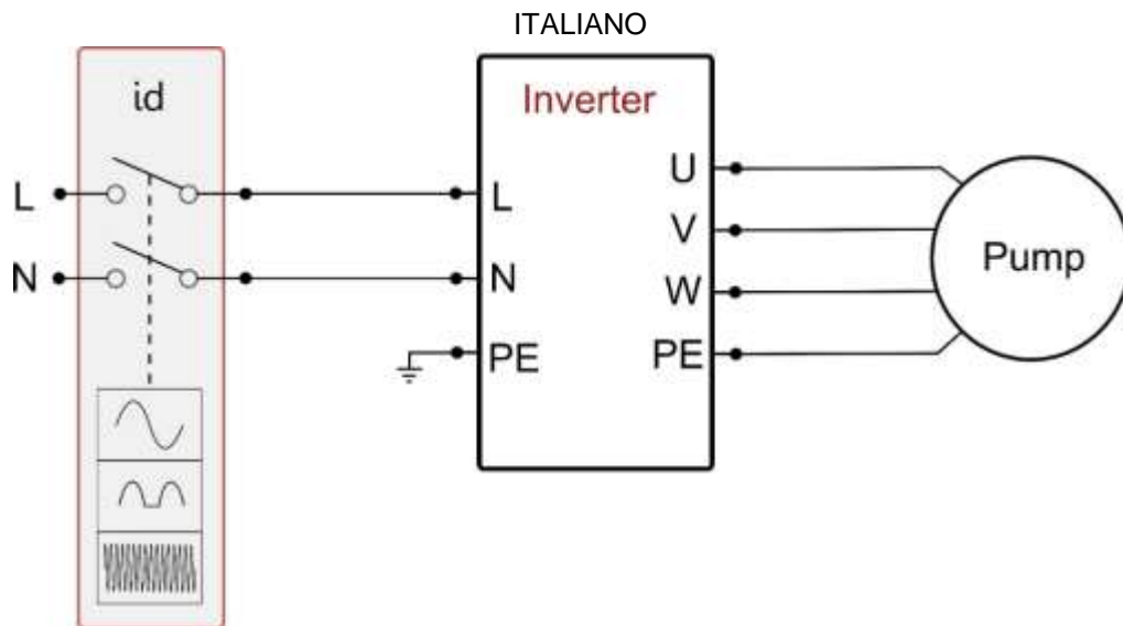
Figura 2a: Esempio di installazione con alimentazione monofase
