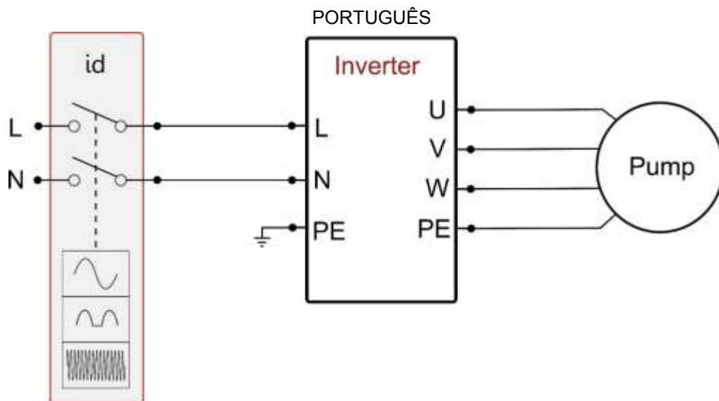
Figura 2a: Exemplo de instalação com alimentação monofásica
