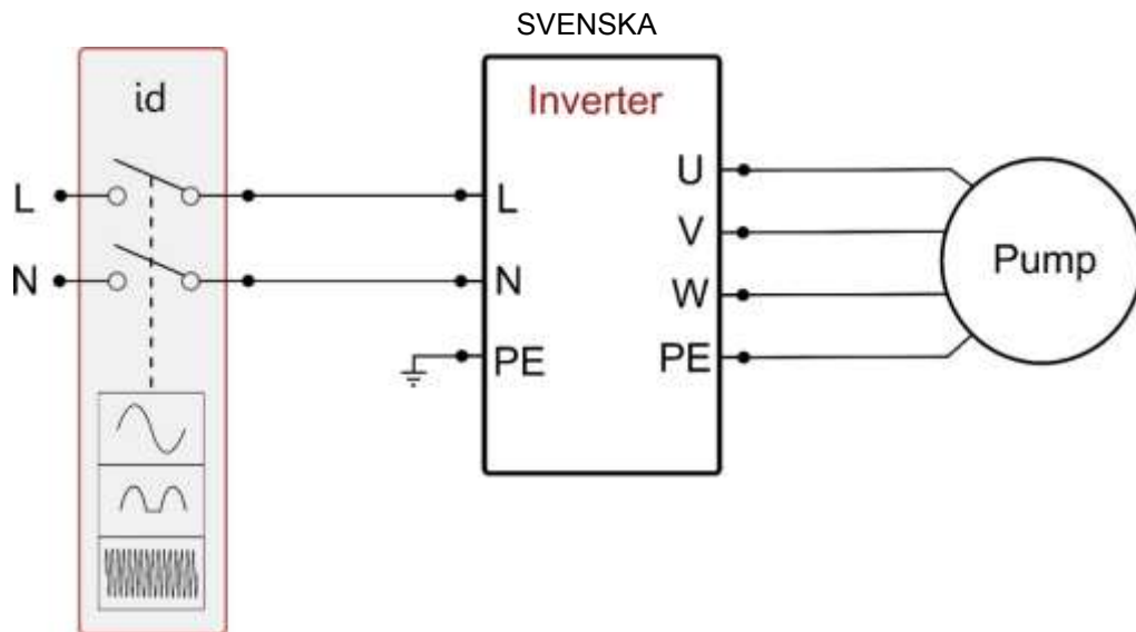
Fig. 2a: Exempel på installation med enfasmatning
