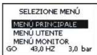
Kuva 12: Alasvetovalikoiden valinta
