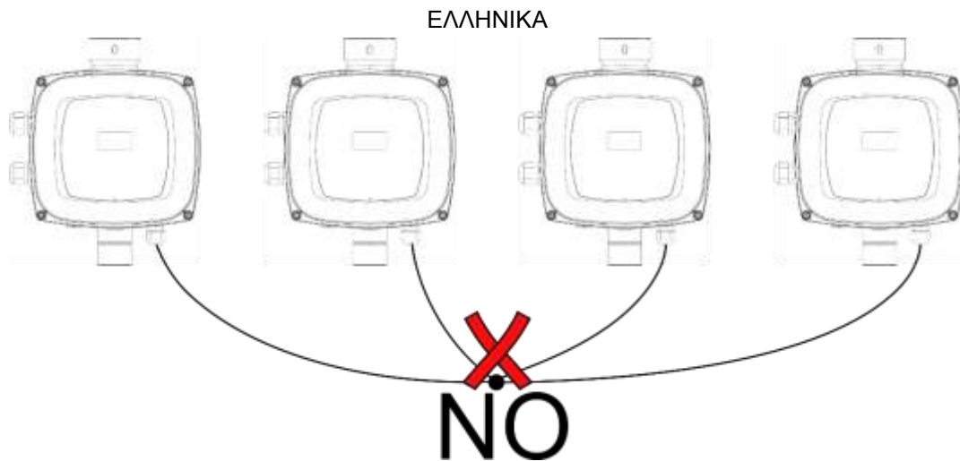
Σχήμα 8: Μην κάνετε σύνδεση αστέρα
