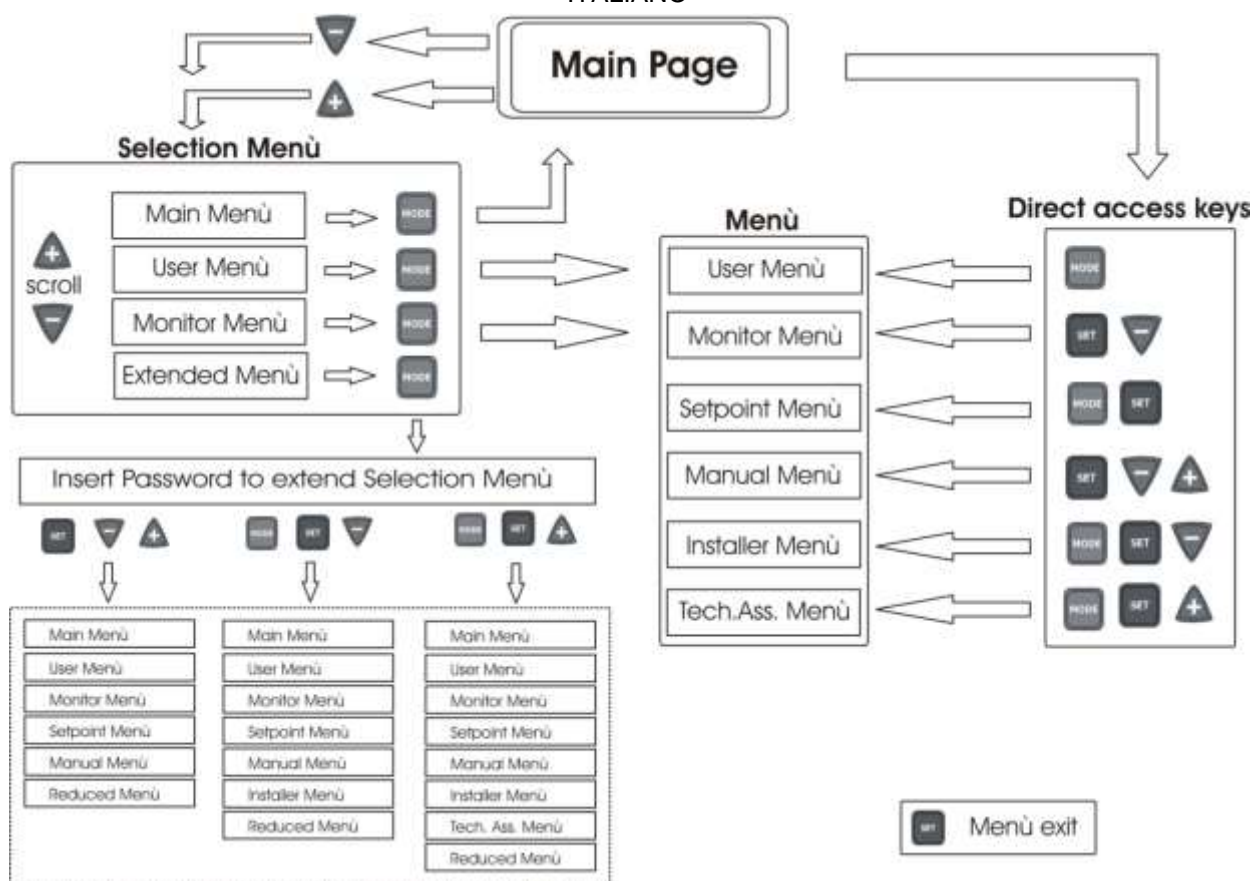
Figura 13: Schema dei possibili accessi ai menù
