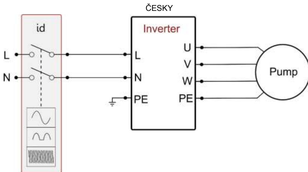
Obr. 2a: Příklad montáže s monofázovým napájením
