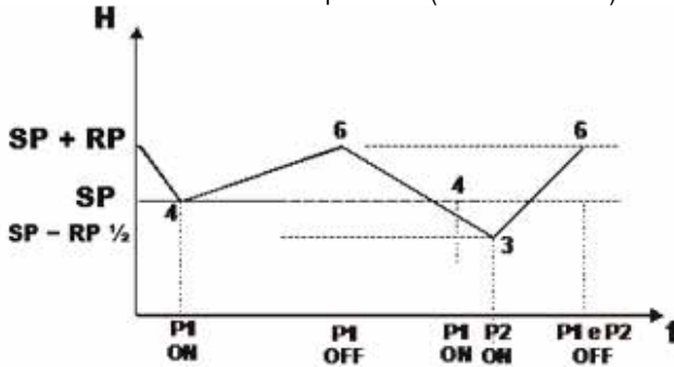
Figura 17: Regolazione con vaso di espansione < 100 litri
