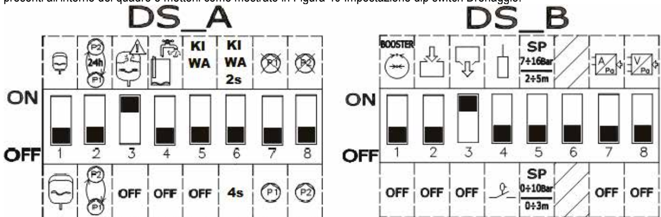
Figura 40: Impostazione dip switch Drenaggio
