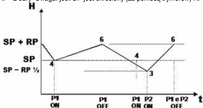
Rysunek 17: Regulacja z naczyniem zbiorczym < 100 litrów
