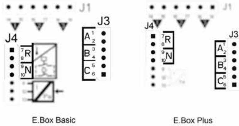
الشكل 20: المداخل ووحدات الحماية
