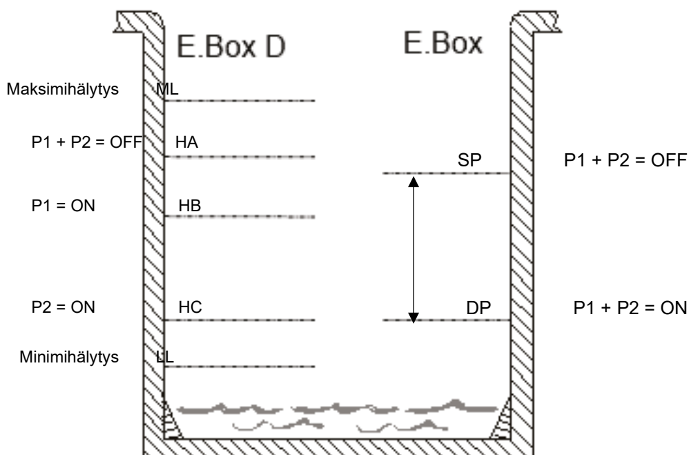
Kuva 30. Täyttö syvyyssanturilla
