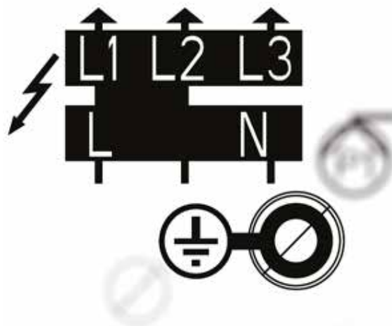
Kuva 5. Sähköverkon liitäntä.
