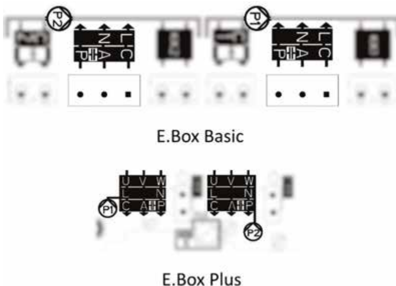
Figura 3: Conexiuni electrice pompe
