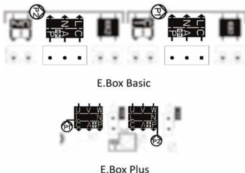
Abbildung 3: Elektroanschlüsse der Pumpen
