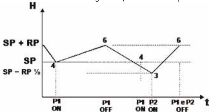
6 Figura 17: Regulación con vaso de expansión < 100 litros FUNCIÓN DE LLENADO
