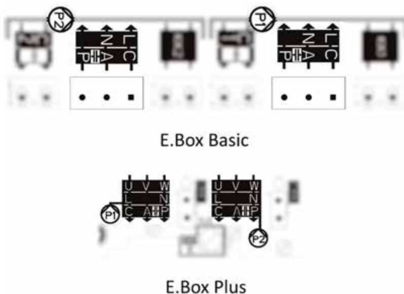
3.ábra: A szivattyúk elektromos bekötése
