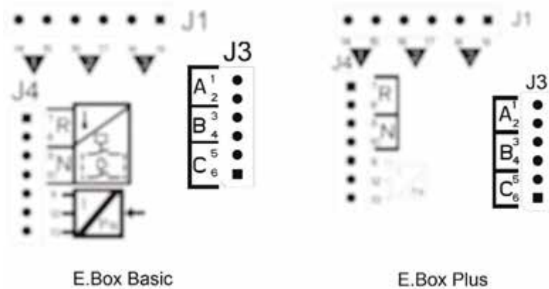
Kuva 11. Painekatkaisimien liittimet
