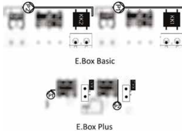
الشكل 33: مداخل الحماية الحرارية KK
