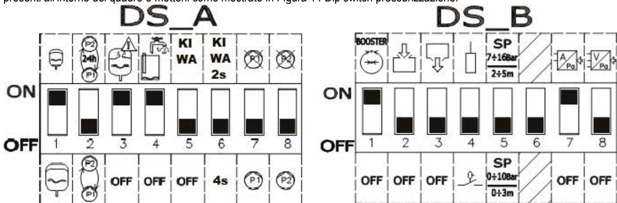
Figura 14: Dip switch pressurizzazione
