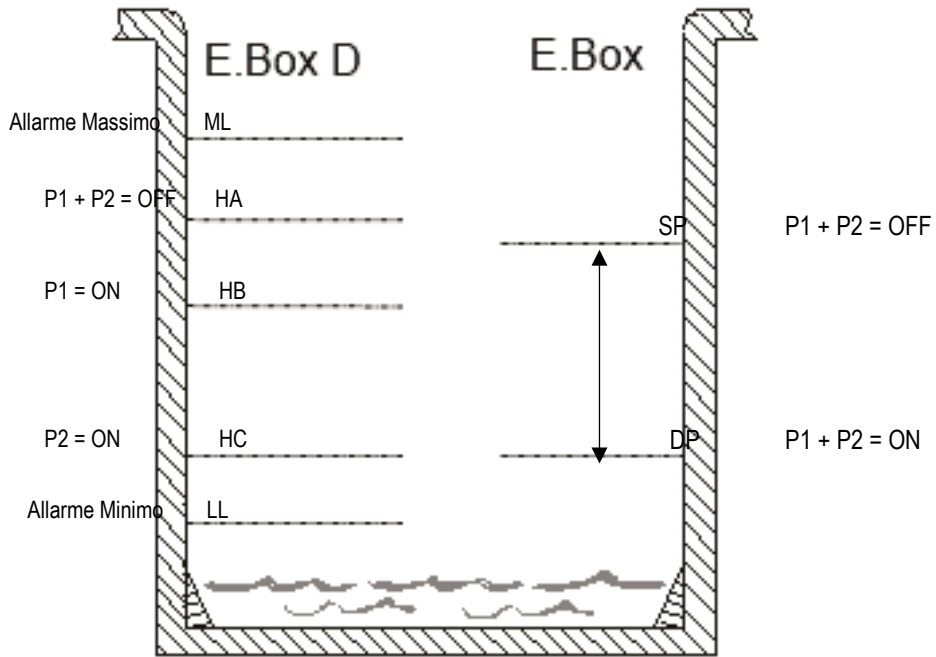
Figura 30: Riempimento con sensore di profondità
