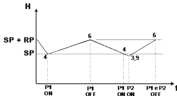
Rysunek 18: Regulacja z naczyniem zbiorczym > 100 litrów
