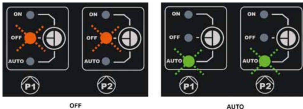
Obrázek 15: Povolení P1 a P2.
