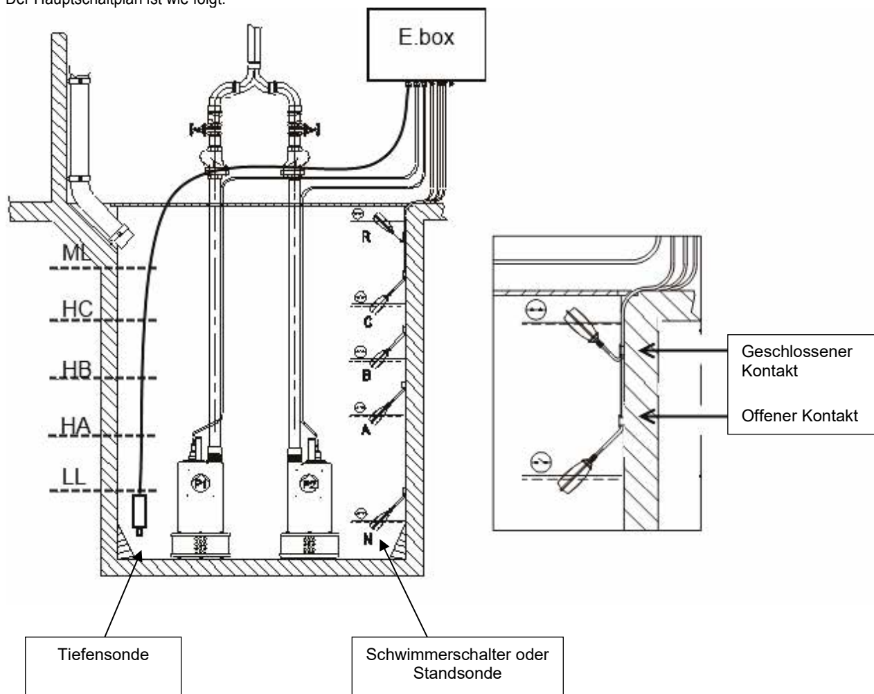
Abbildung 31: Drainage Anlagen-Schaltplan
