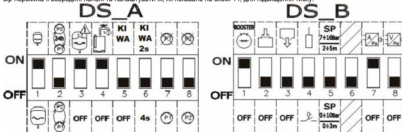
Схема 14: Діп-перемикачі для підвищення тиску
