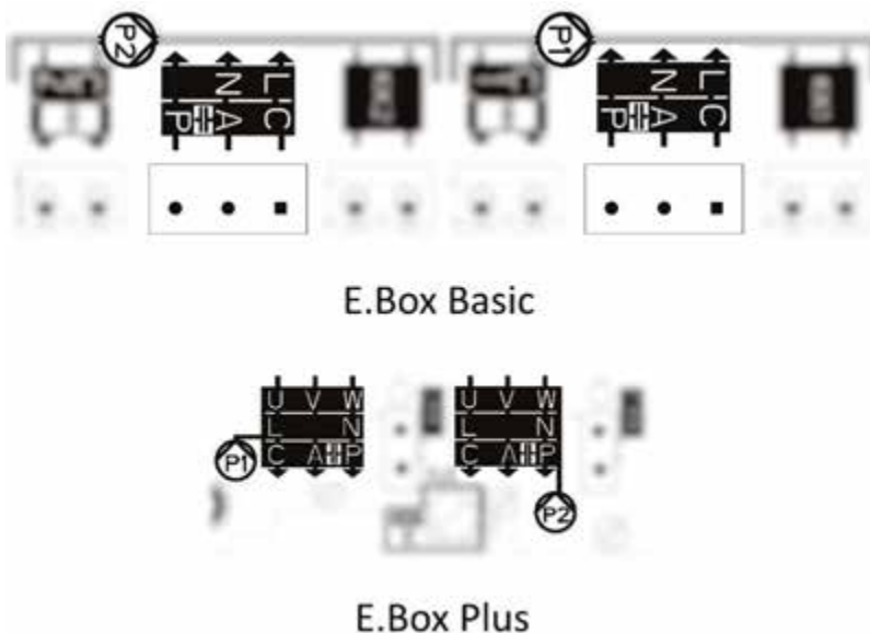
Rysunek 3: Elektryczne podłączenie pomp
