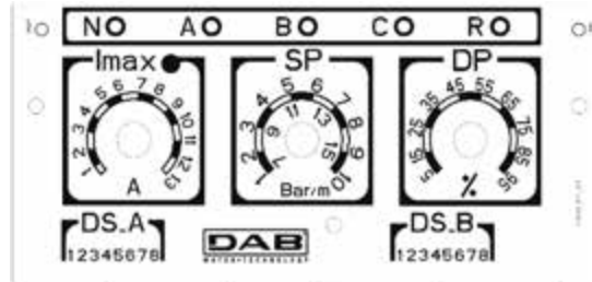
الشكل 16: الضبط: Imax و SP و DP
