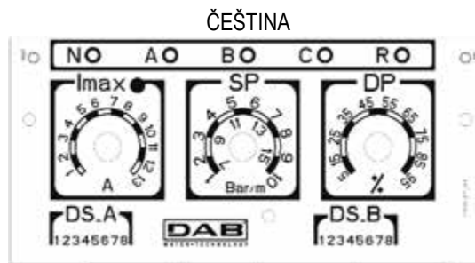
Obrázek 29: Regulování jmenovitého proudu SP a DP
