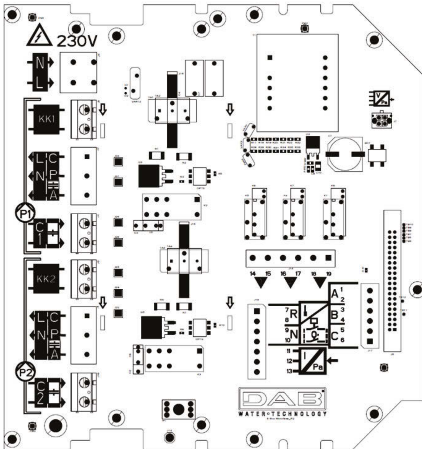
Obrázek 1: Základní deska EBOXU Basic
