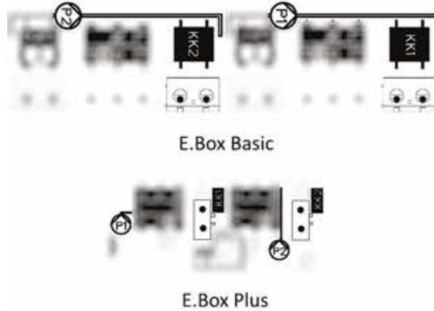
الشكل 45: مداخل الحماية الحرارية KK
