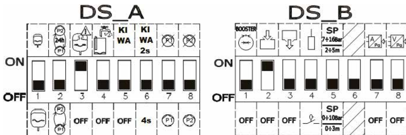
27.ábra: A Dip Switch-ek beállítása a konfigurációhoz
