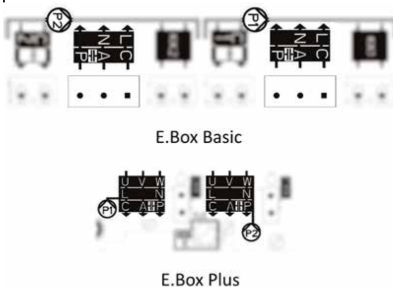
Figura 3: Collegamenti elettrici pompe
