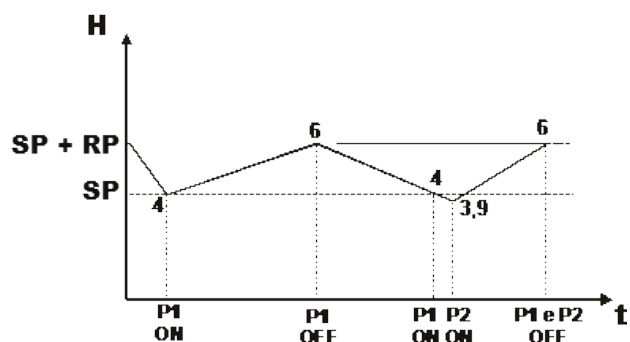
Rysunek 55: Regulacja z naczyniem wzbiorczym > 100 litrów
