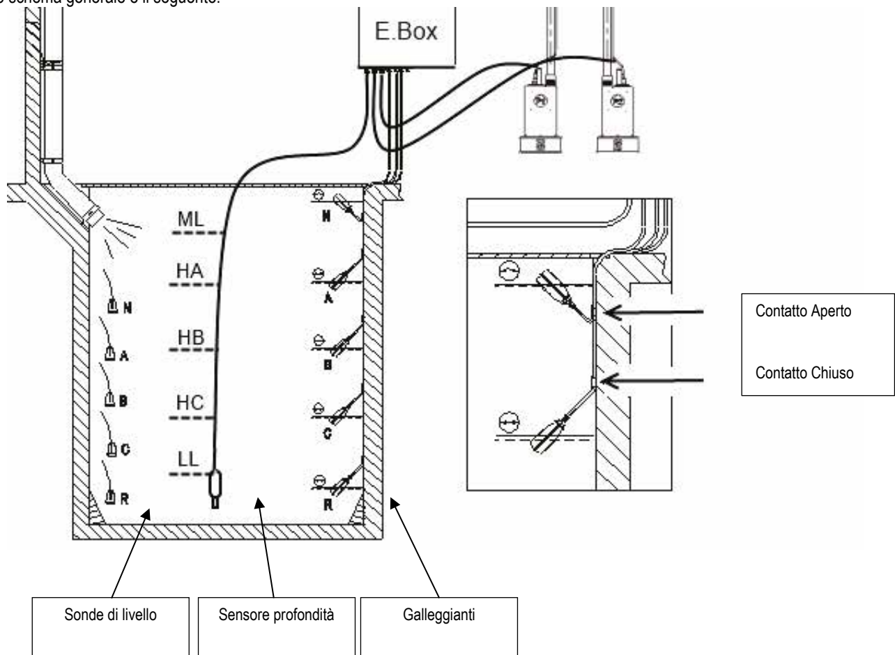
Figura 19: Schema ingressi sistema di riempimento
