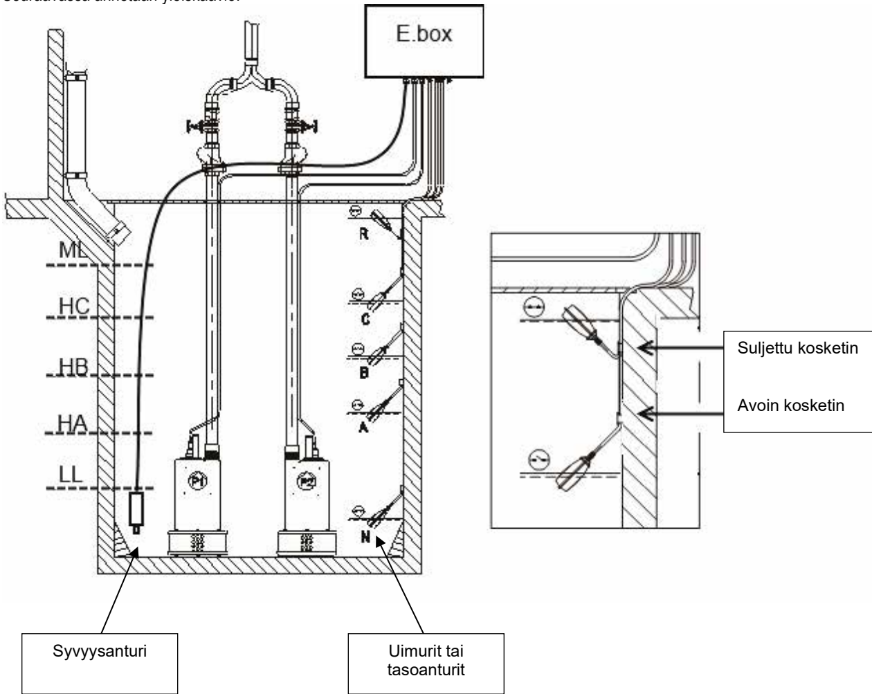
Kuva 31. Tyhjennysjärjestelmän kaavio
