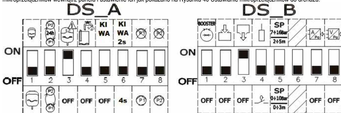
Rysunek 40: Ustawianie mikroprzełączników Drenażu
