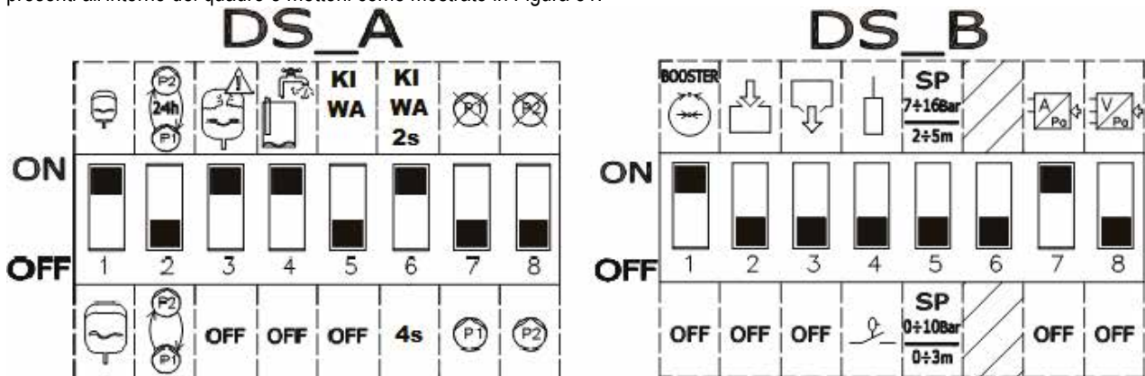
Figura 51: Dip switch pressurizzazione KIWA
