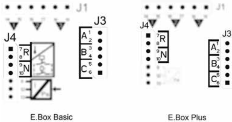
الشكل 8: المداخل والمخارج
