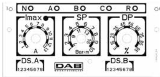
Figure 42 : Réglage du courant nominal SP et DP
