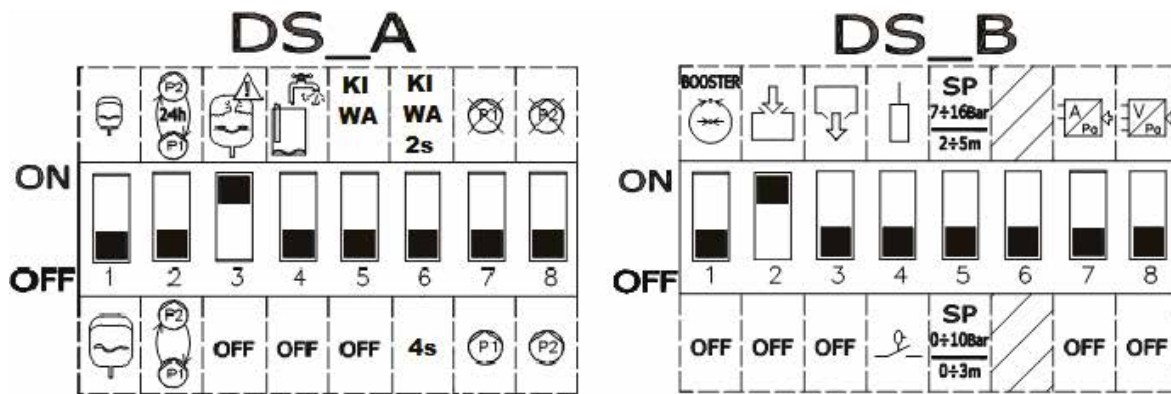
Figura 27: Impostazione dip switch riempimento
