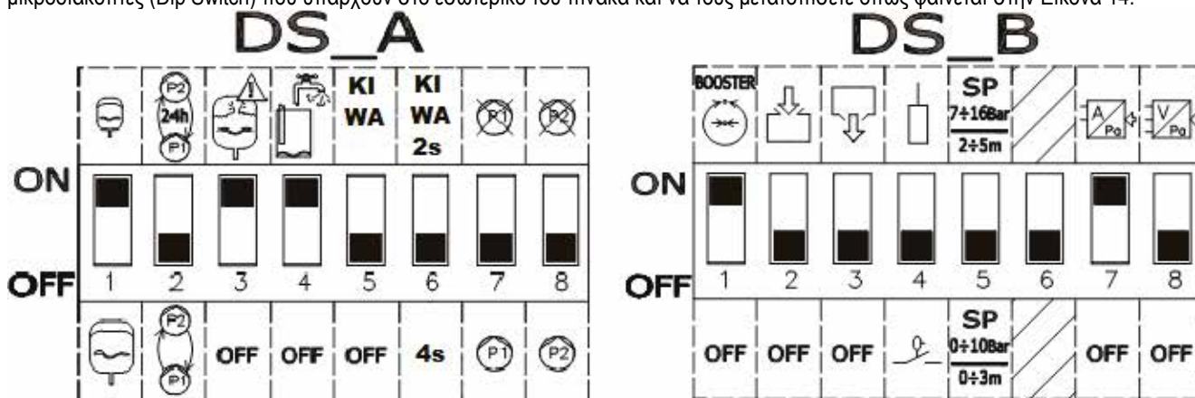
Εικόνα 14: Μικροδιακόπτες (Dip switch) για δημιουργία πίεσης
