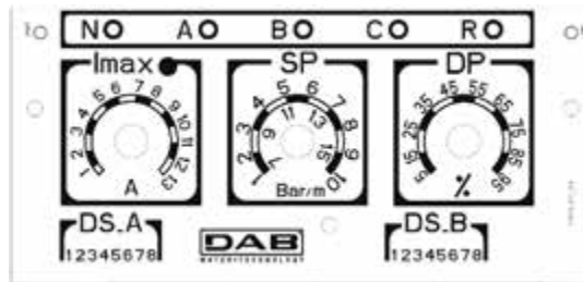
Afbeelding 29: Regeling nominale stroom SP en DP
