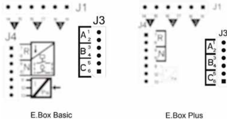
Figura 47: Morsettiera pressostati
