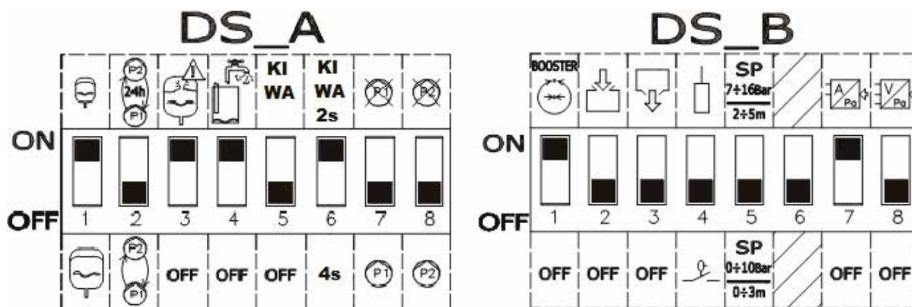
Kuva 51. Dip-kytkimet KIWA-paineistuksessa
