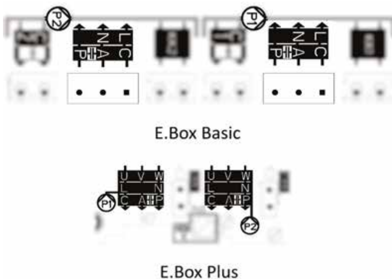
Схема 3: Електричні з'єднання насосів
