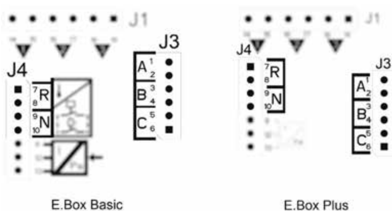
Εικόνα 8: Είσοδοι και έξοδοι
