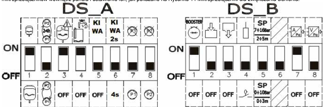
Rysunek 14: Mikroprzełączniki dla zwiększania ciśnienia
