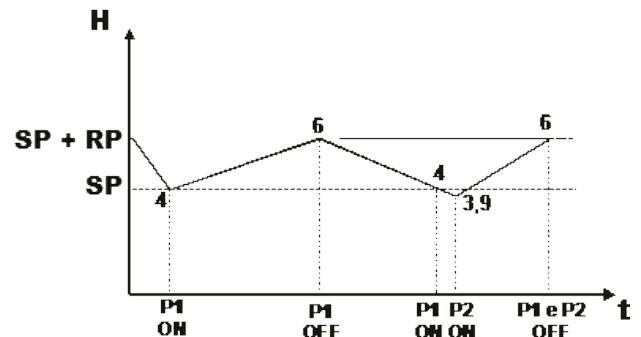
Figure 17 : Réglage avec vase d'expansion supplémentaire &gt; 100 litres
