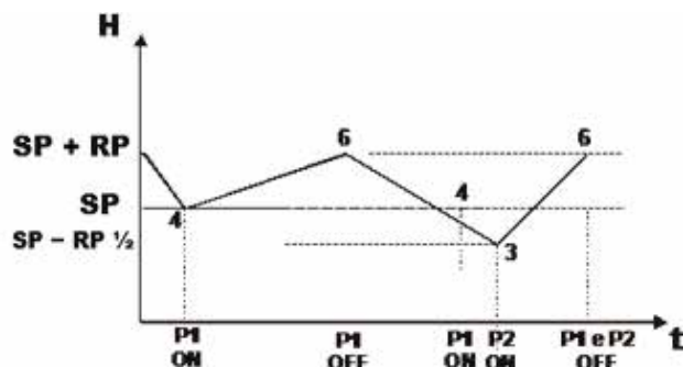
54.ábra: Szabályzás 100 liternél kisebb tágulási tartály esetén
