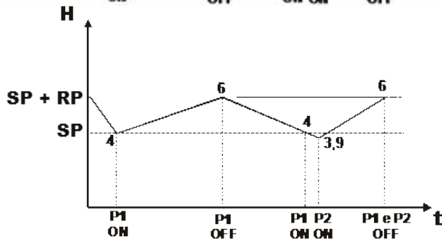
Figura 55: Regolazione con vaso di espansione < 100 litri
