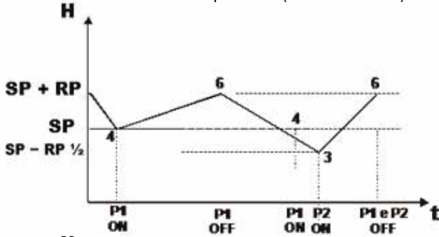
Figura 54: Regolazione con vaso di espansione < 100 litri
