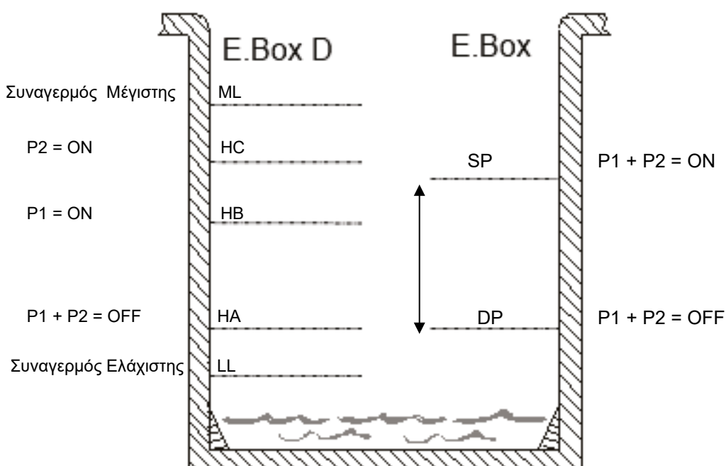
Εικόνα 43: Εκκίνηση με αισθητήρα βάθους
