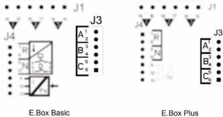
Kuva 47. Paineatkaisimien liitinalusta
