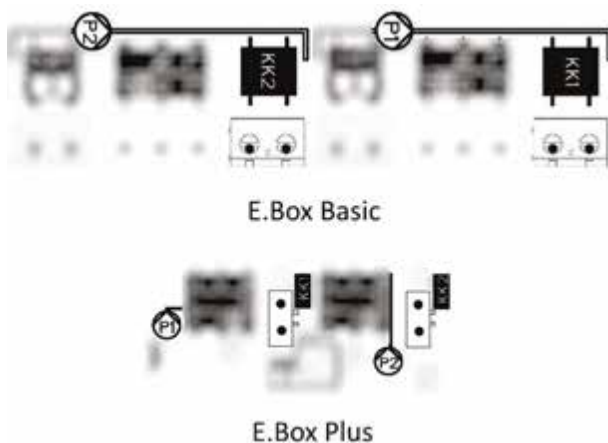
Εικόνα 45: Είσοδοι θερμικής προστασίας KK
