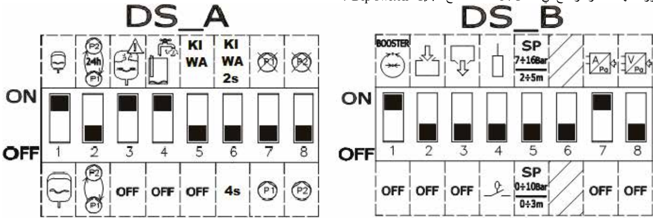
الشكل 14: ضغط مفتاح التبديل "Dip switch"
