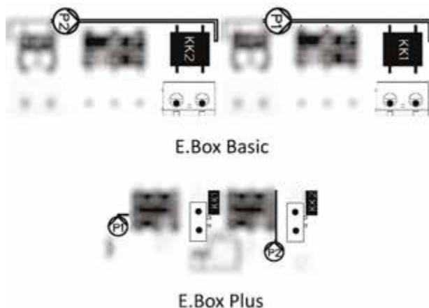
21.ábra: A motor hővédelmének bemenete: KK jelű sorkapocs
