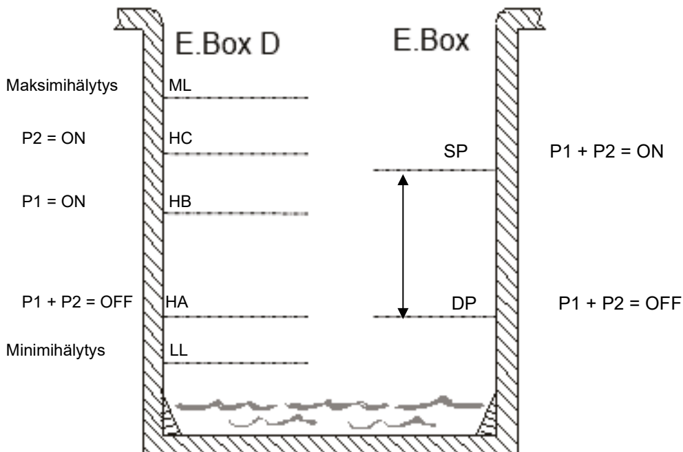
Kuva 43. Tyhjennys syvyyssanturilla
