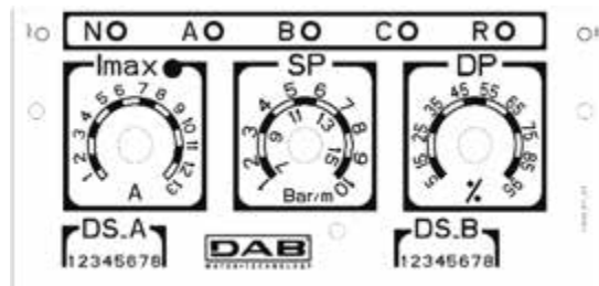
Figura 16: Reglare: I max , SP și DP
