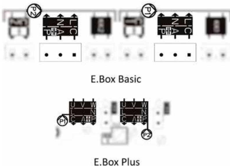
Εικόνα 3: Ηλεκτρική συνδεσμολογία αντλιών
