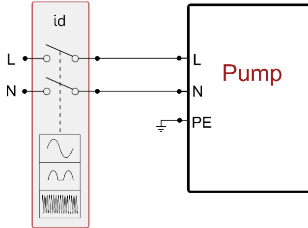
Slika 10 Primer instalacije
