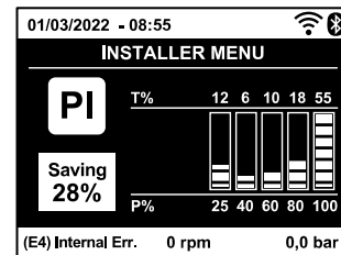
Kuva 17.2: Tehohistogrammin näyttö (3) (4)
