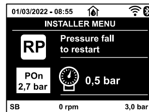
Kuva 18.2: Uudelleenkäynnistyspaineen asetukset (3) (4)
