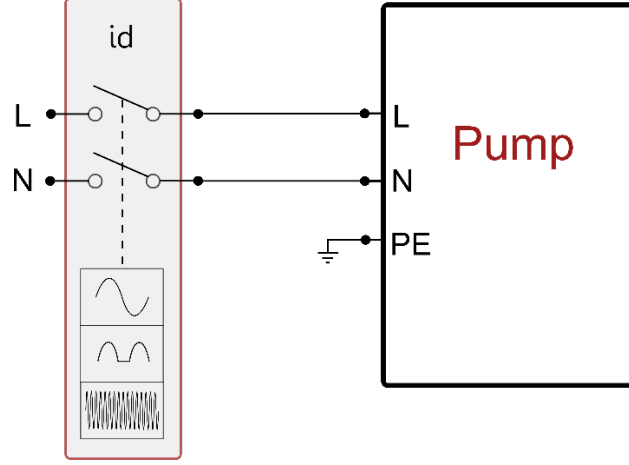
Şekil 10 Montaj Örneği
